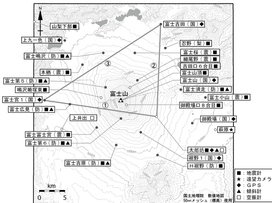
図 5 富士山 観測点配置図
