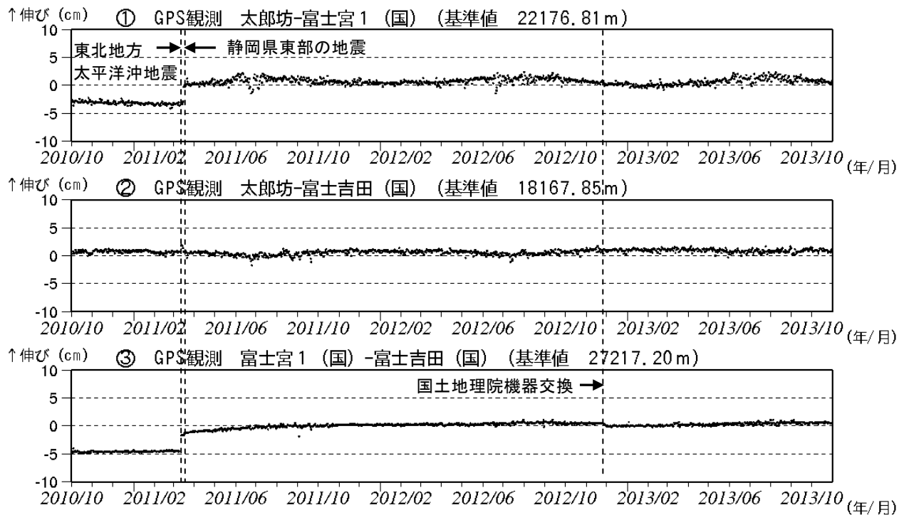
図 4 富士山 GPS 連続観測による基線長変化（2010 年 10 月 1 日～2013 年 10 月 31 日）
