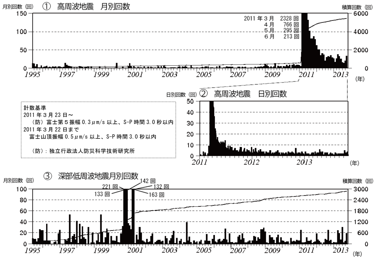
図 2 富士山 月別及び日別地震回数（1995 年 6 月～2013 年 10 月）
