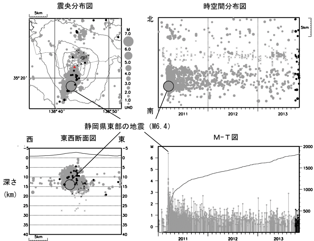
図 3 富士山 広域地震観測網による山体・周辺の地震活動（2011 年 1 月 1 日～2013 年 10 月 31 日）
