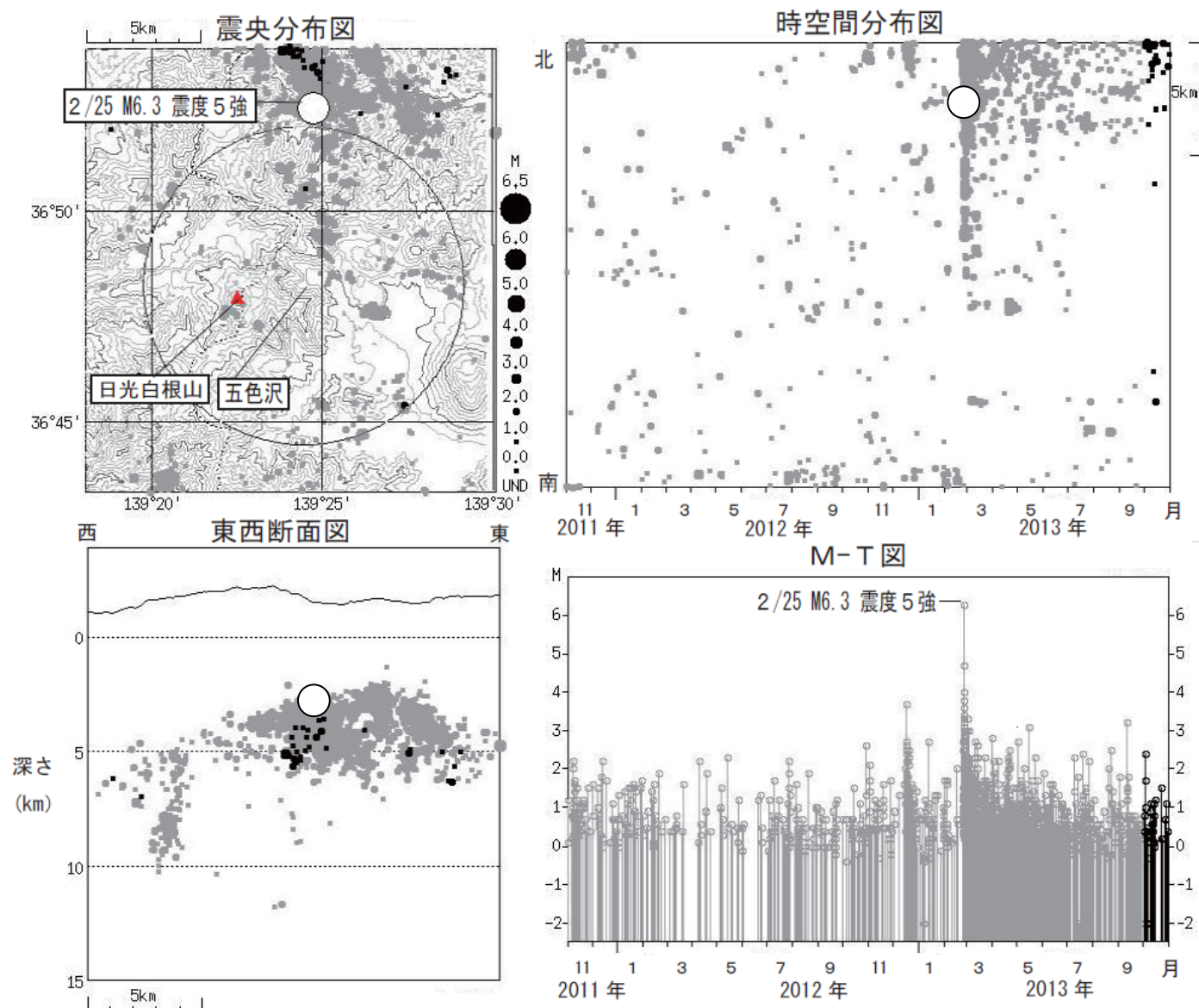
図3 日光白根山 広域地震観測網による山体・周辺の地震活動(2011年11月1日～2013年10月31日)
