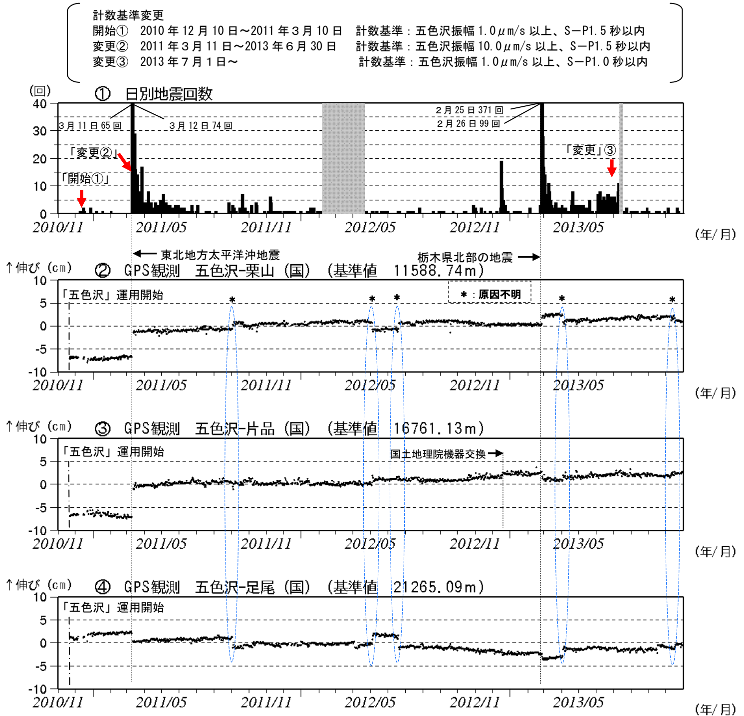
図2 日光白根山 火山活動経過図 (2010 年 11 月 20 日～2013 年 10 月 31 日)
