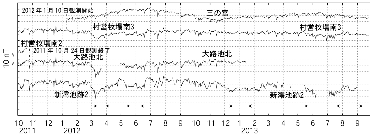
図 6 三宅島 全磁力連続観測による全磁力値の変化（2011 年 10 月～2013 年 9 月） 基準点：雄山北東
