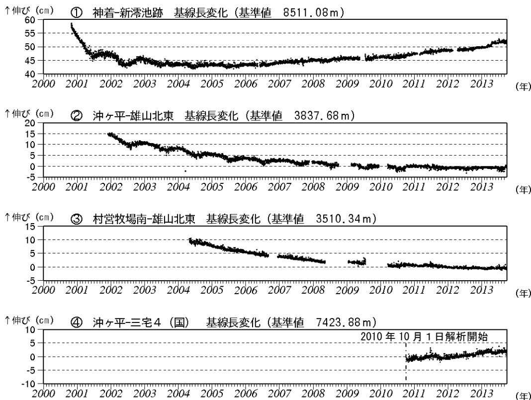
図 5 三宅島 GPS 連続観測結果（2000 年 1 月～2013 年 9 月）（国）：国土地理院 ・基線①～④は図 9（観測点配置図）の①～④にそれぞれ対応します。 ・グラフの空白部分は欠測を示します。 ・2010 年 10 月以降のデータについては、電離層の影響を補正する等、解析方法を改良しています。
