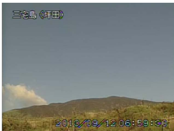
図 1 三宅島 山頂火口からの噴煙の状況 （9月12日、坪田遠望カメラによる）
