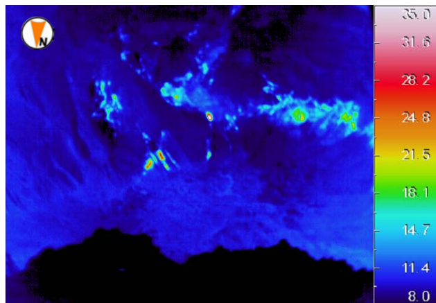
図 3 三宅島 山頂火口南側内壁に位置する主火孔の状況と地表面温度分布 1) 前回の観測（2013年2月20日）と比べ、大きな変化は認められませんでした。
