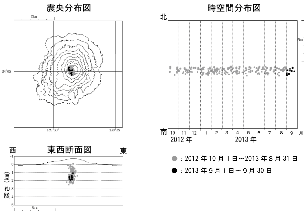
図 7 三宅島 震源分布図（2012 年 10 月 1 日～2013 年 9 月 30 日）
