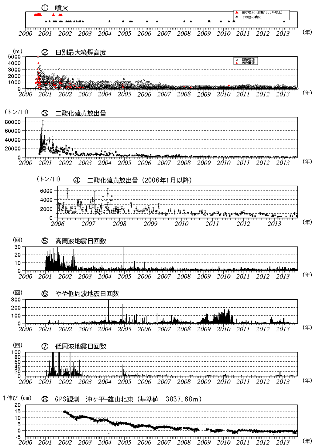
図 4 三宅島 最近の火山活動の経過図（2000 年 1 月～2013 年 9 月）
