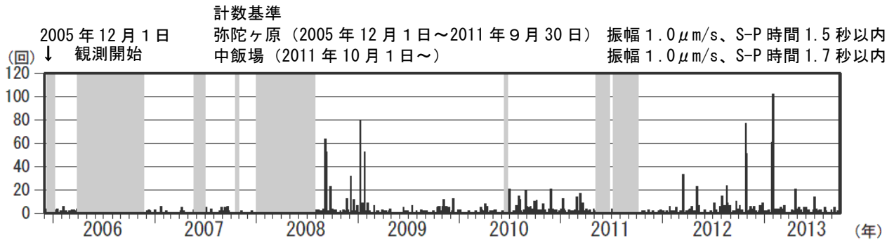
図 3 白山 日別地震回数（2005 年 12 月～2013 年 9 月）
