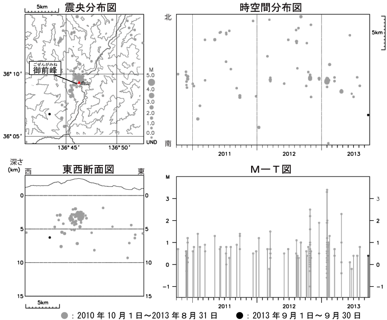
図 4 白山 広域地震観測網による山体・周辺の地震活動（2010 年 10 月 1 日～2013 年 9 月 30 日）
