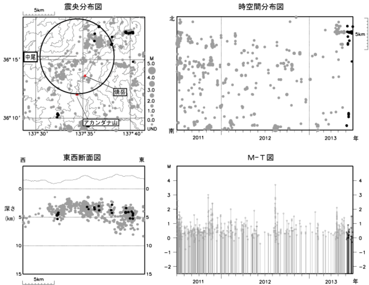
図4 焼岳 広域地震観測網による山体・周辺の地震活動(2011年7月1日～2013年6月30日)
