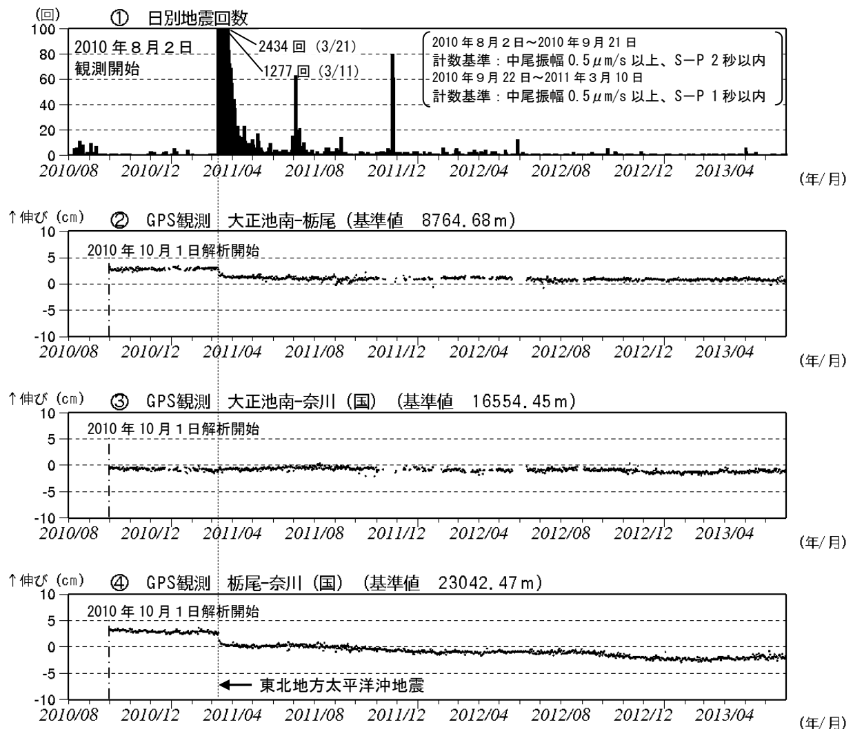
図 3 焼岳 火山活動経過図（2010 年 8 月 2 日～2013 年 6 月 30 日）
