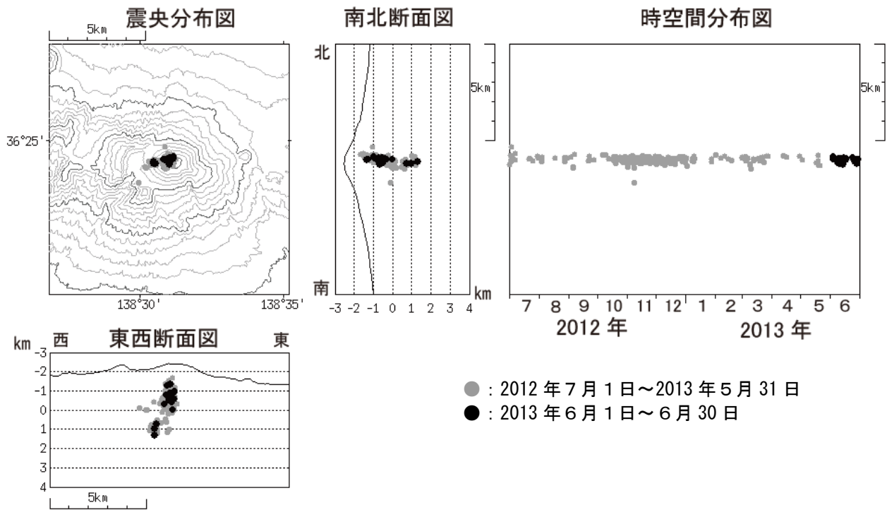
図 4 浅間山 震源分布図（2012 年 7 月 1 日～2013 年 6 月 30 日）
