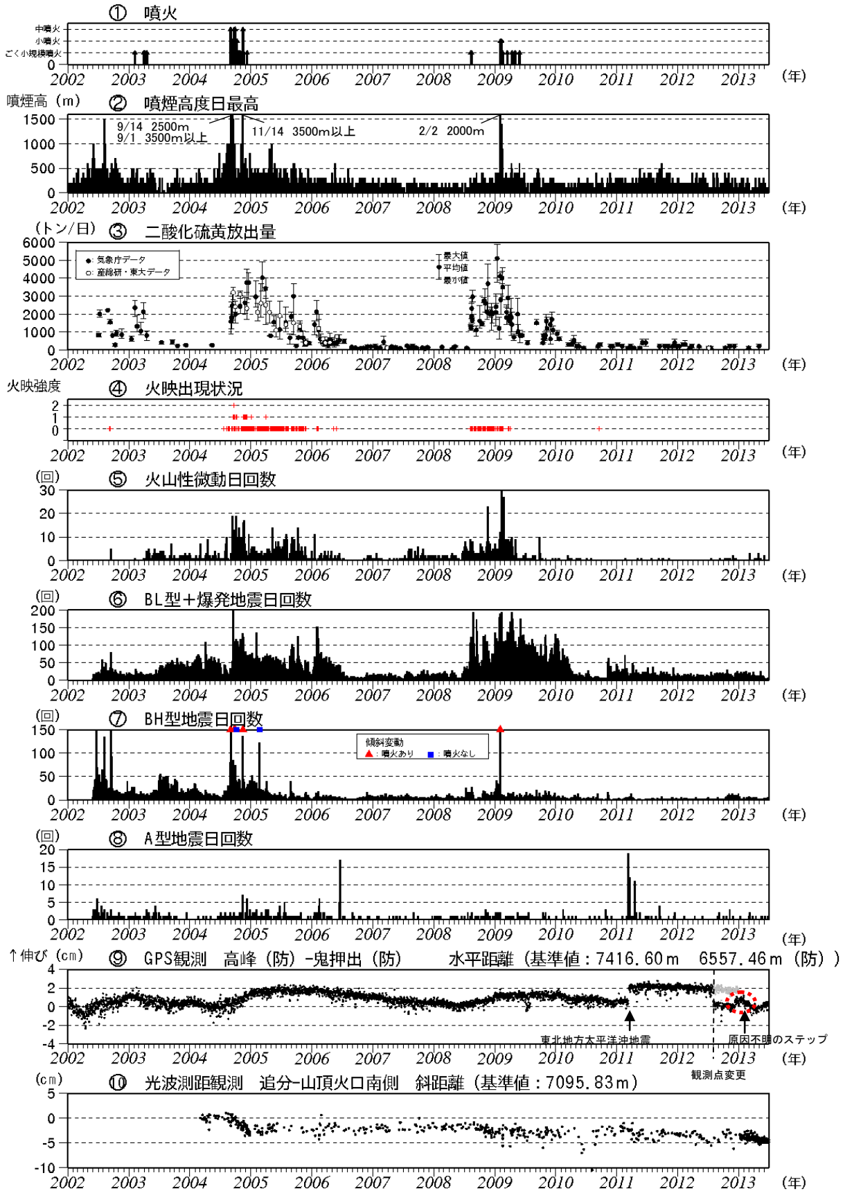
図3 浅間山 最近の火山活動経過図 (2002年1月1日~2013年6月30日)
