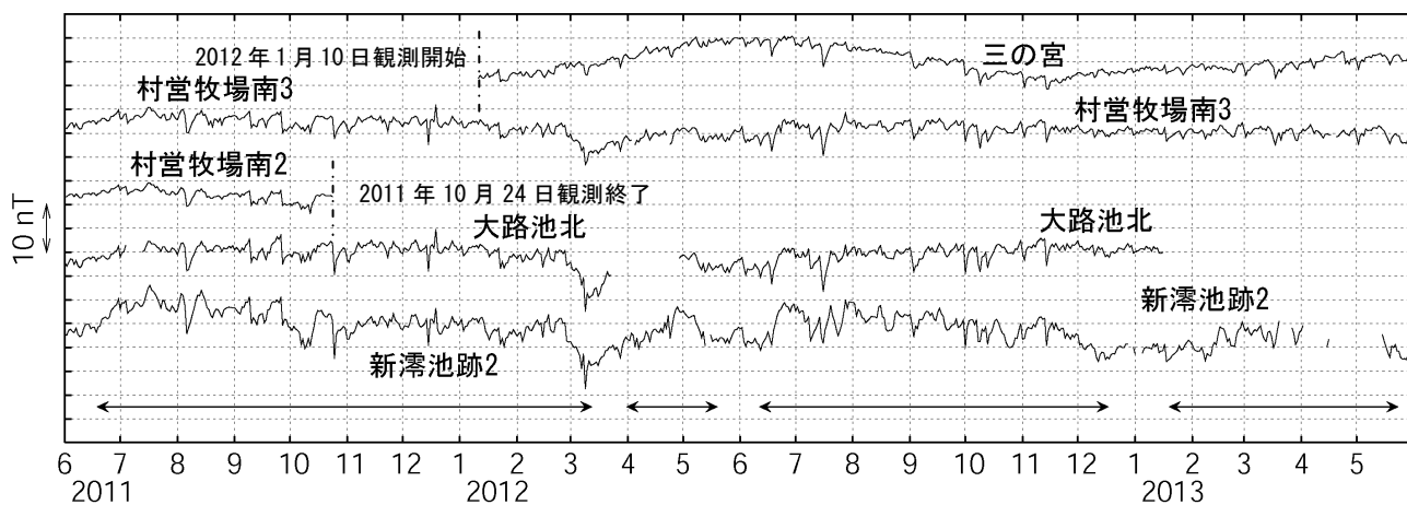
図4 三宅島 全磁力連続観測による全磁力値の変化 (2011年6月～2013年5月) 基準点：雄山北東
