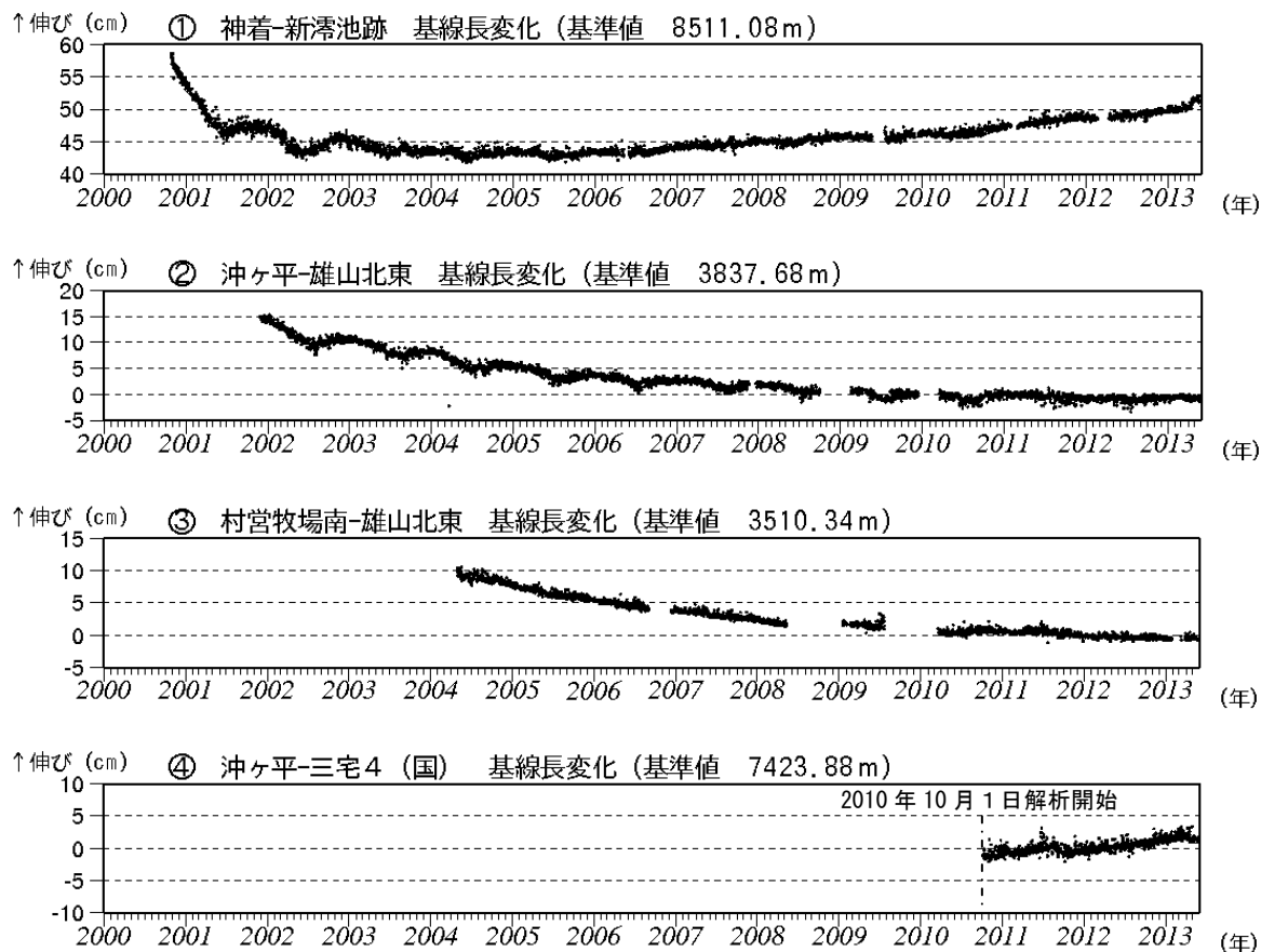
図3 三宅島 GPS 連続観測結果 (2000年1月～2013年5月) (国)：国土地理院 ・基線①～④は図7（観測点配置図）の①～④にそれぞれ対応します。 ・グラフの空白部分は欠測を示します。 ・2010年10月以降のデータについては、電離層の影響を補正する等、解析方法を改良しています。
