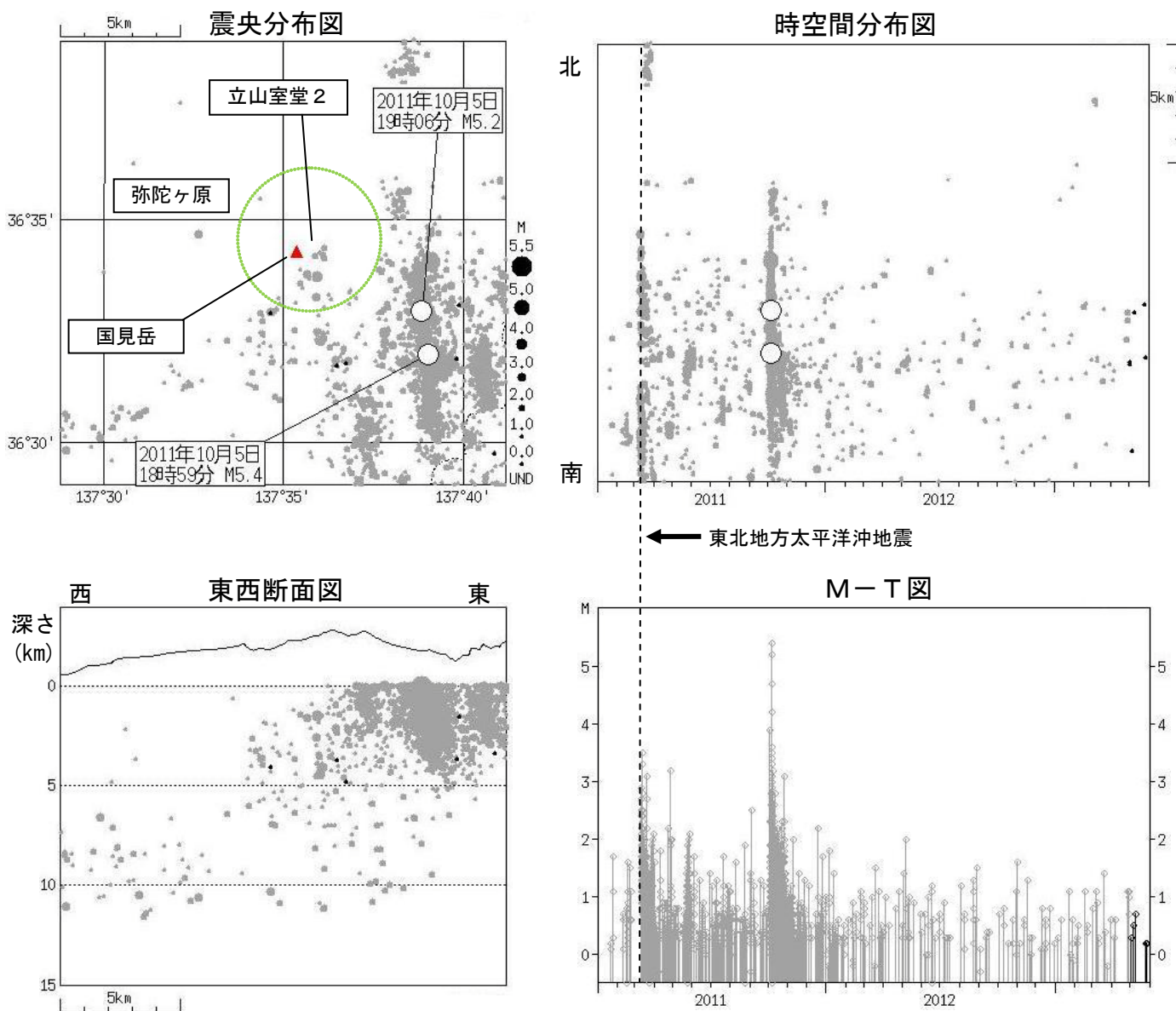
図 2 弥陀ヶ原 広域地震観測網による山体・周辺の地震活動 (2011 年 1 月 1 日～2013 年 5 月 31 日)
