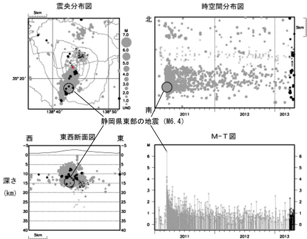
図 3 ※ 富士山 広域地震観測網による山体・周辺の地震活動 (2011 年 1 月 1 日～2013 年 4 月 30 日)
