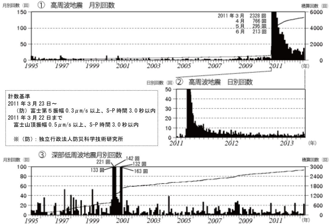
図 2 ※ 富士山 月別及び日別地震回数 (1995 年 6 月～2013 年 4 月)
