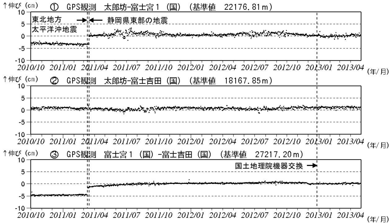
図 4 ※ 富士山 GPS 連続観測による基線長変化（2010 年 10 月 1 日～2013 年 4 月 30 日）
