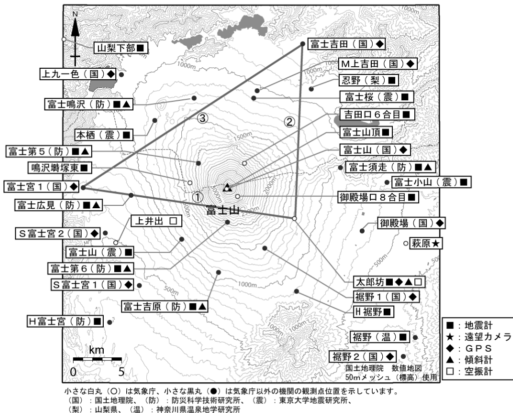
図 5 富士山 観測点配置図 GPS 基線①～③は図 4 ※の①～③に対応しています。
