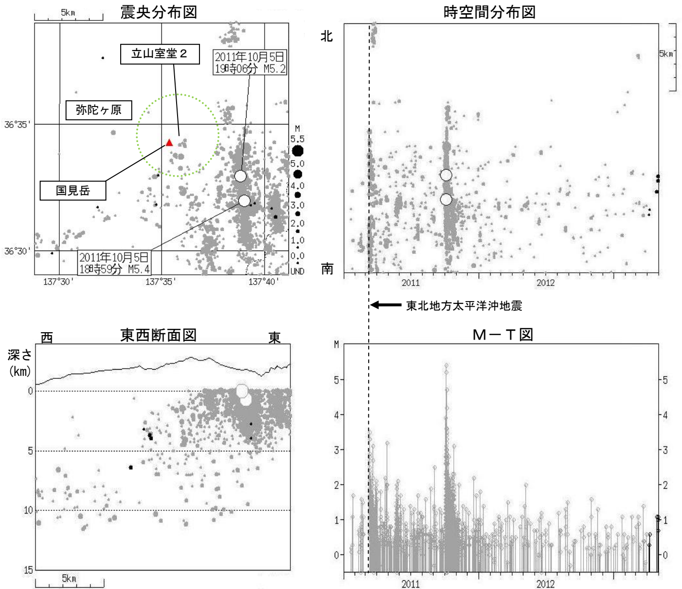
図 2※ 彌陀ヶ原 広域地震観測網による山体・周辺の地震活動 (2011 年 1 月 1 日～2013 年 4 月 30 日) ● : 2011 年 1 月 1 日～2013 年 3 月 31 日 ● : 2013 年 4 月 1 日～4 月 30 日 ・ 緑色の点線の円は、立山室堂に設置した地震計 (立山室堂 2) で S-P 時間 1 秒以内となるおよそその範囲を示します。 ・ 今期間、周辺の地震活動は低下しながら継続しています。 ・ 彌陀ヶ原近傍の地震活動は、低調な状況で経過しました。 ・ M (マグニチュード) は地震の規模を表します。 ・ 図中の震源要素は一部暫定値が含まれており、後日変更することがあります。
