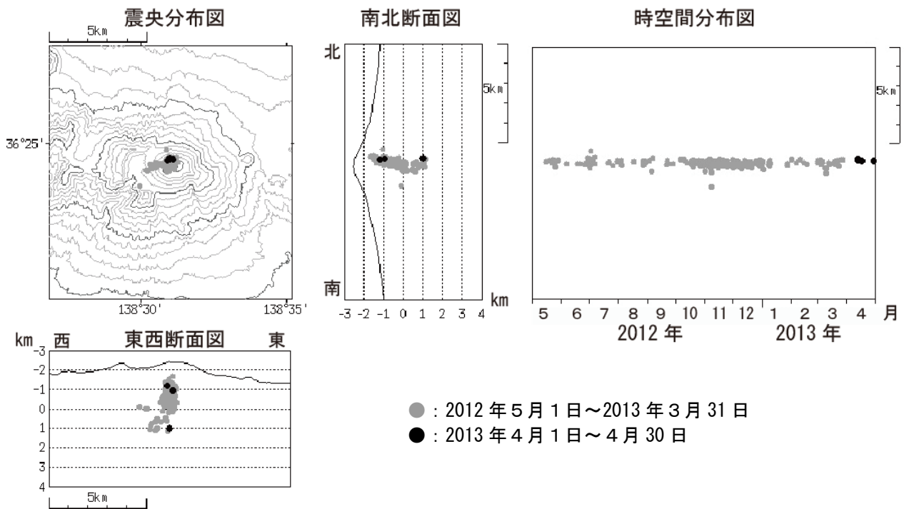
図 4 ※ 浅間山 震源分布図（2012 年 5 月 1 日～2013 年 4 月 30 日）
