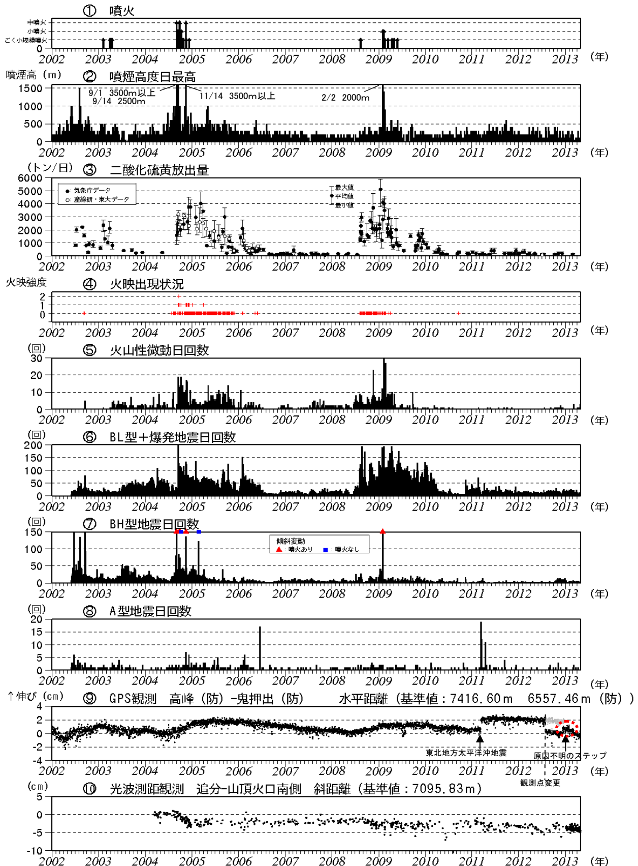
図3※ 浅間山 最近の火山活動経過図(2002年1月1日~2013年4月30日)
