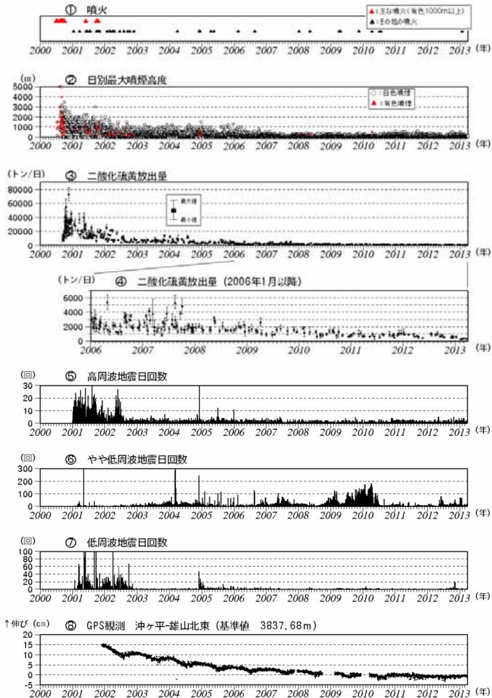
図 2 三宅島 最近の火山活動の経過図（2000 年 1 月～2013 年 3 月）
