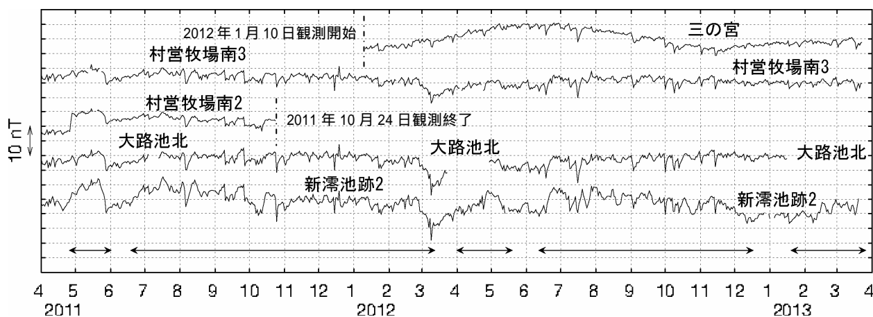
図4 三宅島 全磁力連続観測による全磁力値の変化(2011年4月~2013年3月) 基準点: 雄山北東
