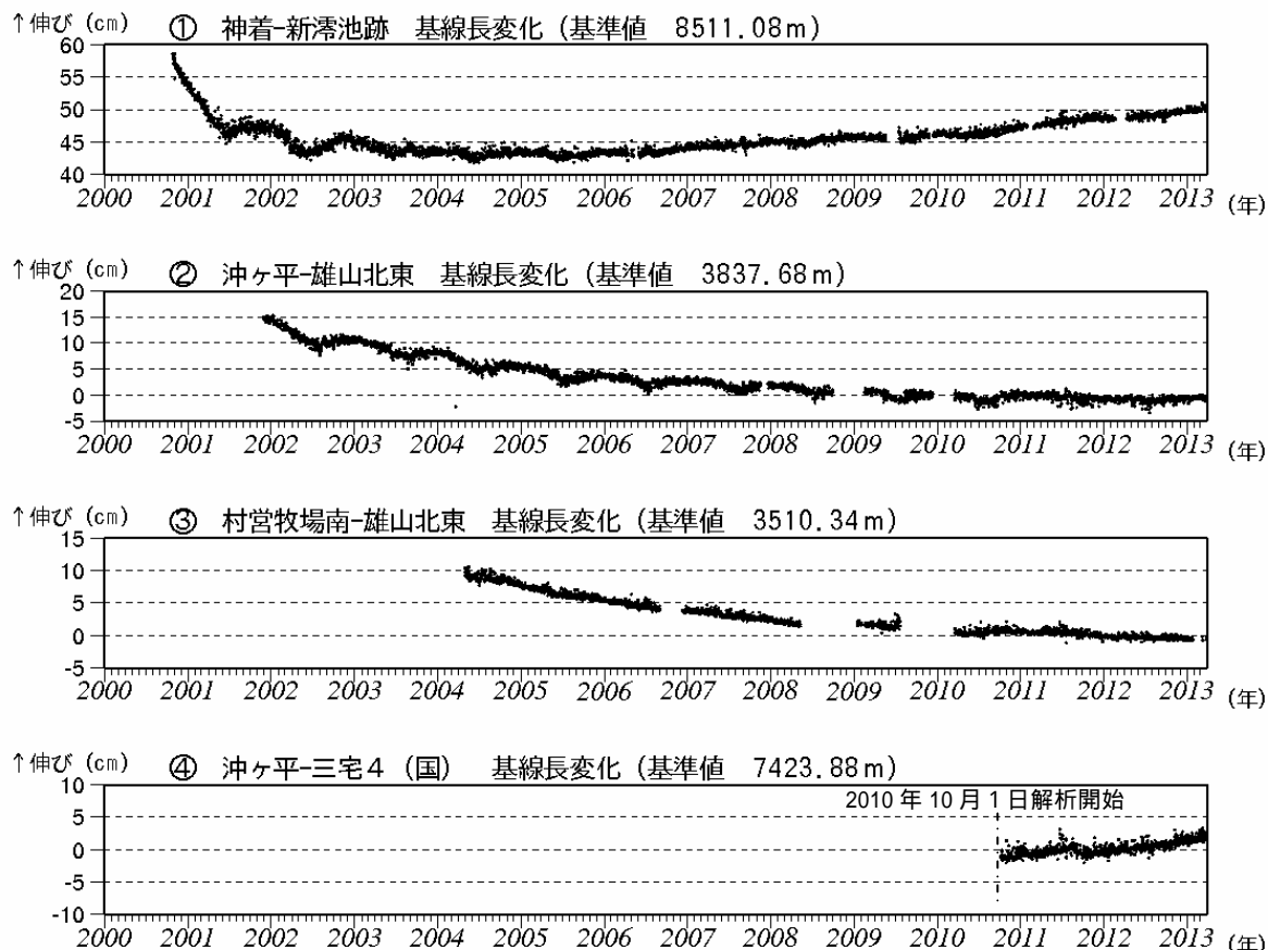
図3 三宅島 GPS連続観測結果(2000年1月~2013年3月) (国): 国土地理院 基線 ~ は図7(観測点配置図)の ~ にそれぞれ対応します。 グラフの空白部分は欠測を示します。 2010年10月以降のデータについては、電離層の影響を補正する等、解析方法を改良しています。
