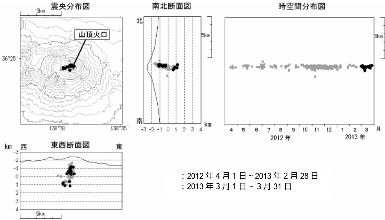
図 4 浅間山 震源分布図(2012 年 4 月 1 日~2013 年 3 月 31 日)
