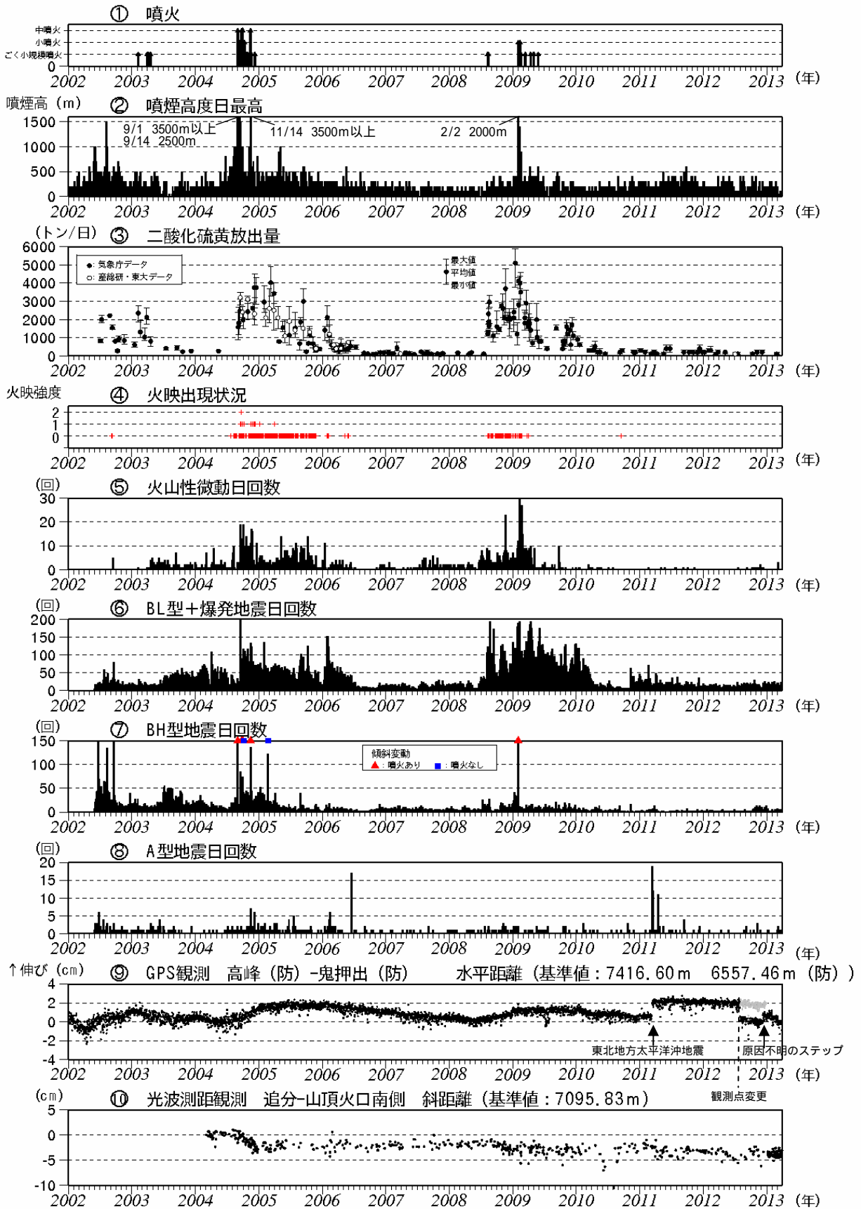
図3 浅間山 最近の火山活動経過図(2002年1月1日~2013年3月31日)
