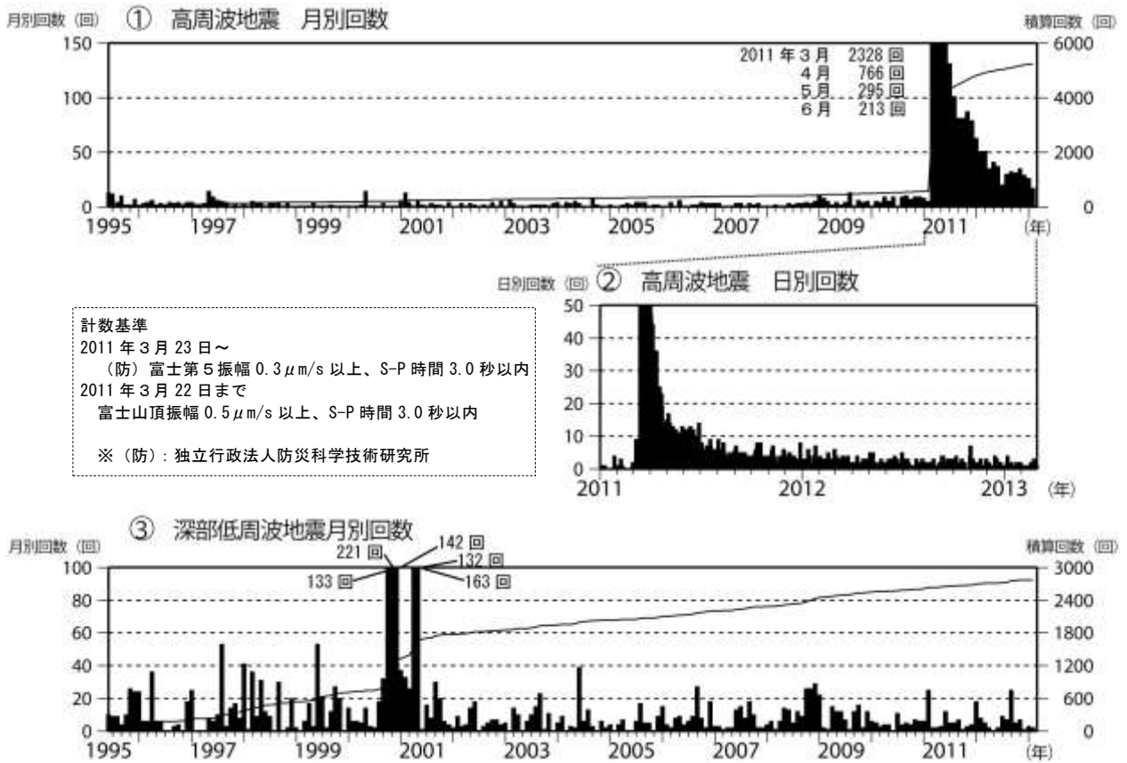
図 2 ※ 富士山 月別及び日別地震回数 (1995 年 6 月～2013 年 2 月)
