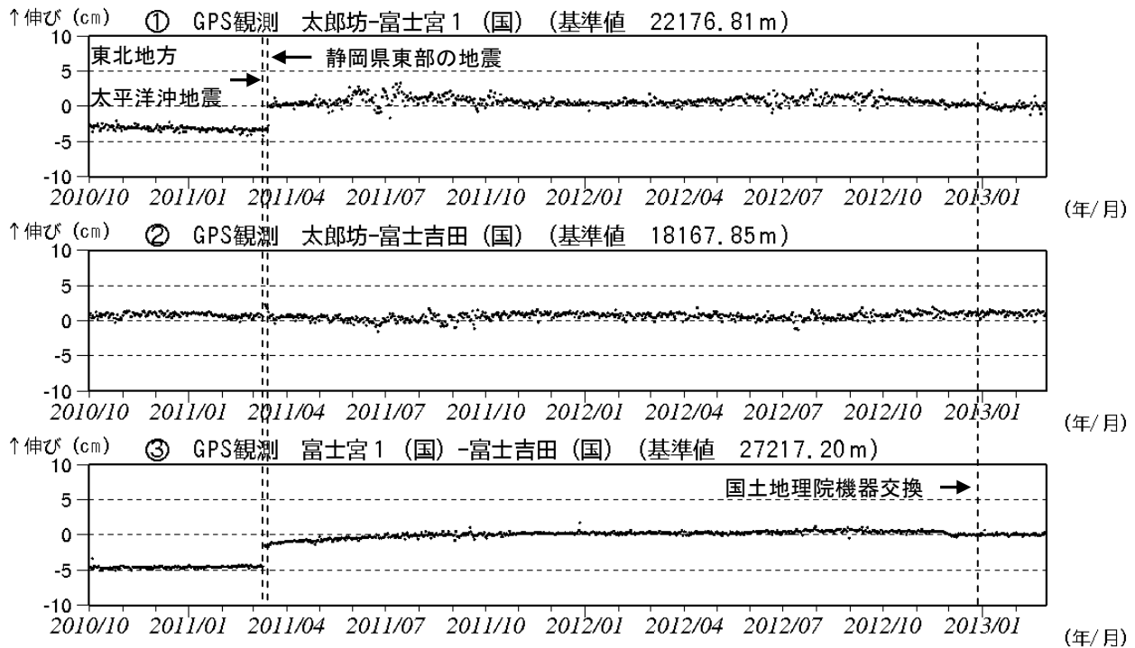
図 4※ 富士山 GPS 連続観測による基線長変化（2010 年 10 月 1 日～2013 年 2 月 28 日）
