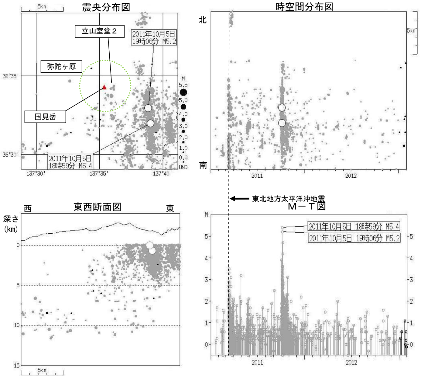
図 2※ 弥陀ヶ原 広域地震観測網による山体・周辺の地震活動（2011 年 1 月 1 日～2013 年 1 月 31 日）
