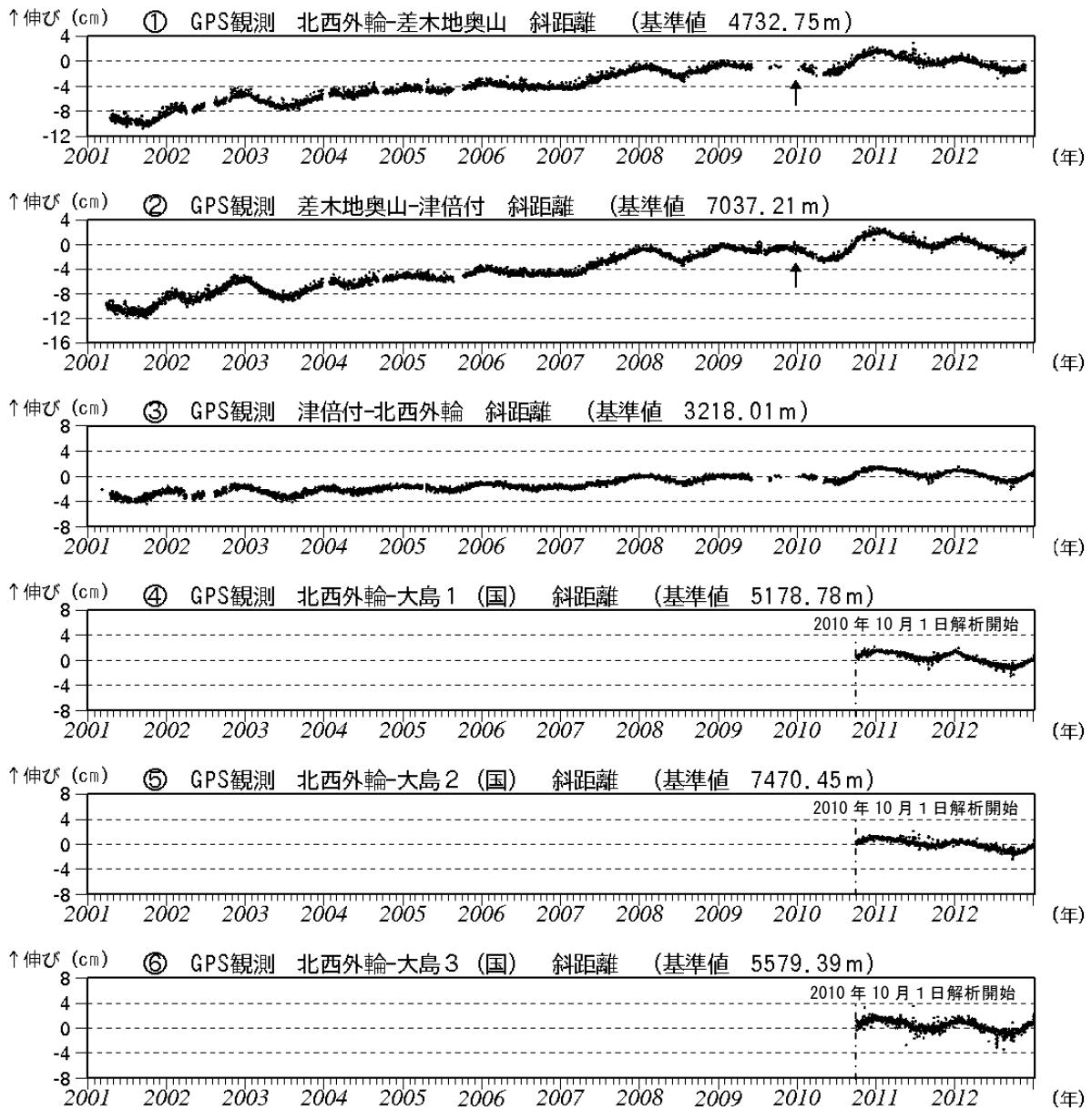
図3※ 伊豆大島 GPS 連続観測による基線長変化 (2001 年 1 月～2012 年 12 月) (国) : 国土地理院 2010 年 10 月以降のデータについては、電離層の影響を補正する等、解析方法を改良しています。 ①～③、及び④※～⑥※は図8のGPS基線①～⑥に対応しています。 グラフの空白部分は欠測。2012 年 11 月 24 日以降、差木地奥山は欠測。 ①②の矢印は差木地奥山支柱工事による変動。
