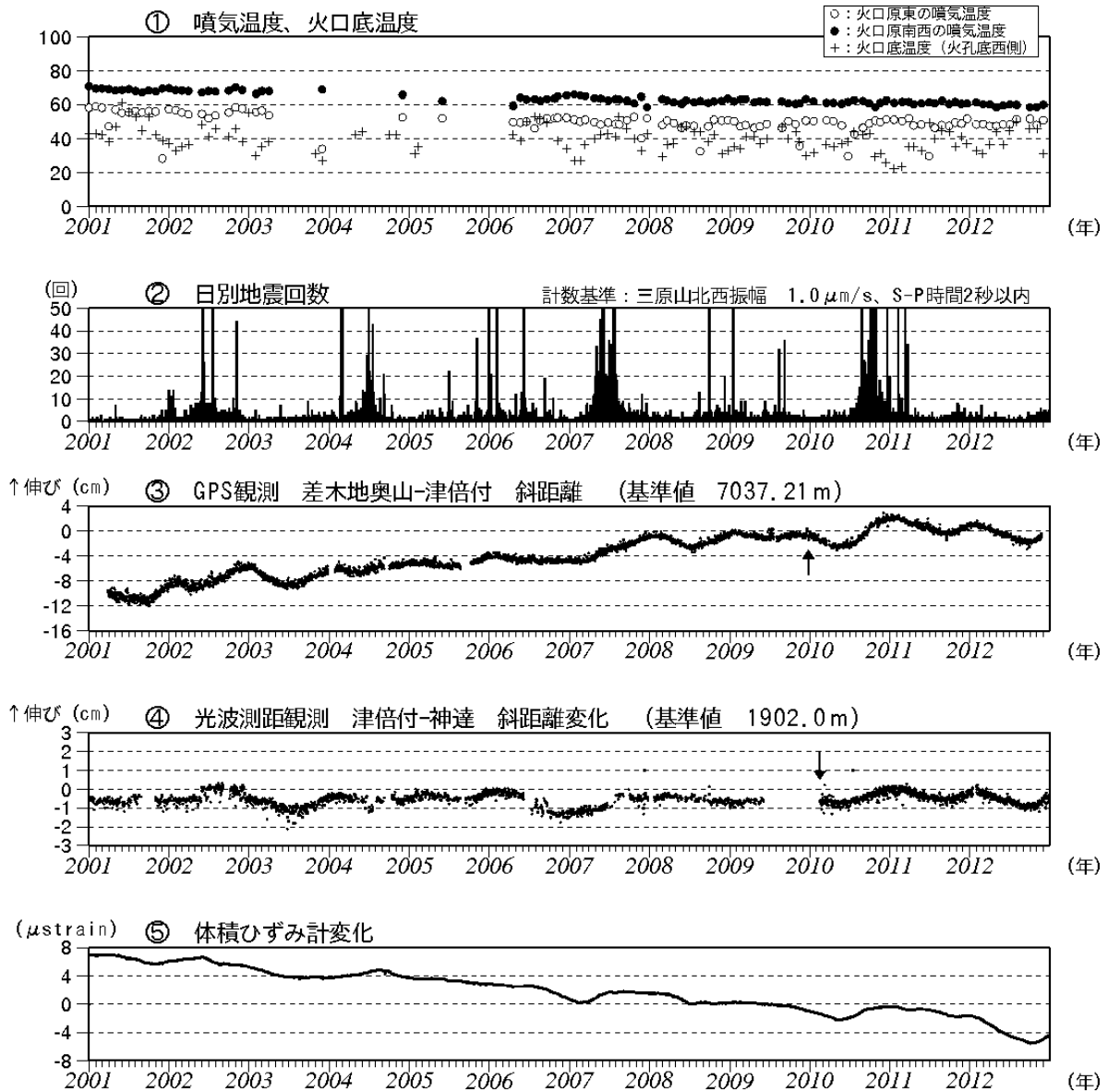
図2 伊豆大島 最近の火山活動経過図 (2001年1月～2012年12月)
