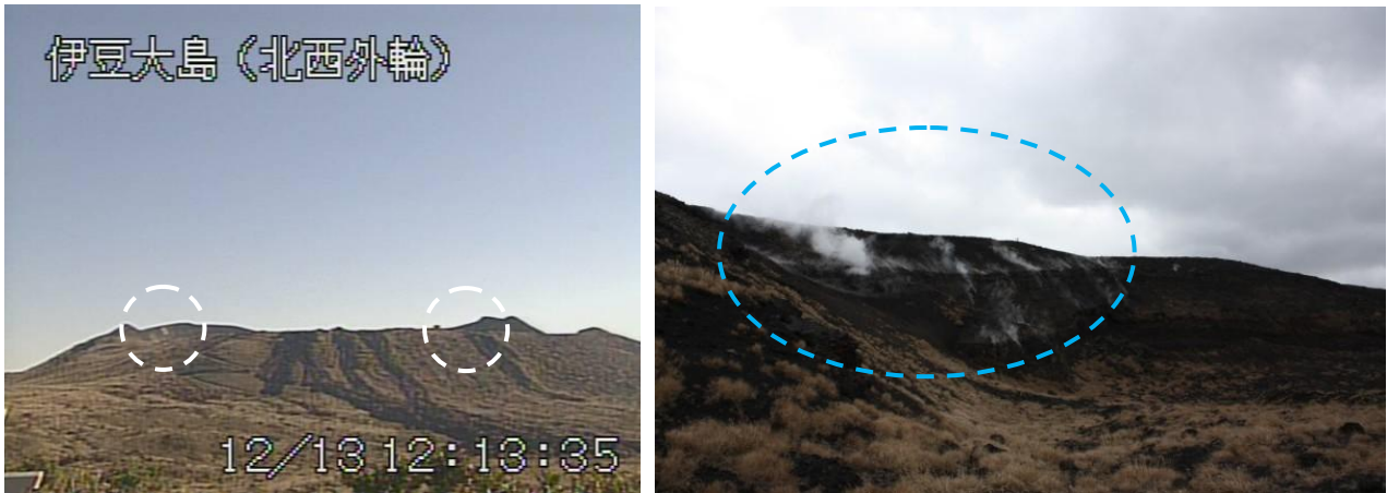
山頂部 (12 月 13 日、北西外輪遠望カメラによる) 剣ガ峰付近 (12 月 21 日、撮影方向は図 6 参照) 図 4 伊豆大島 三原山山頂部及び山頂火口の状況 点円内: ごく弱い噴気
