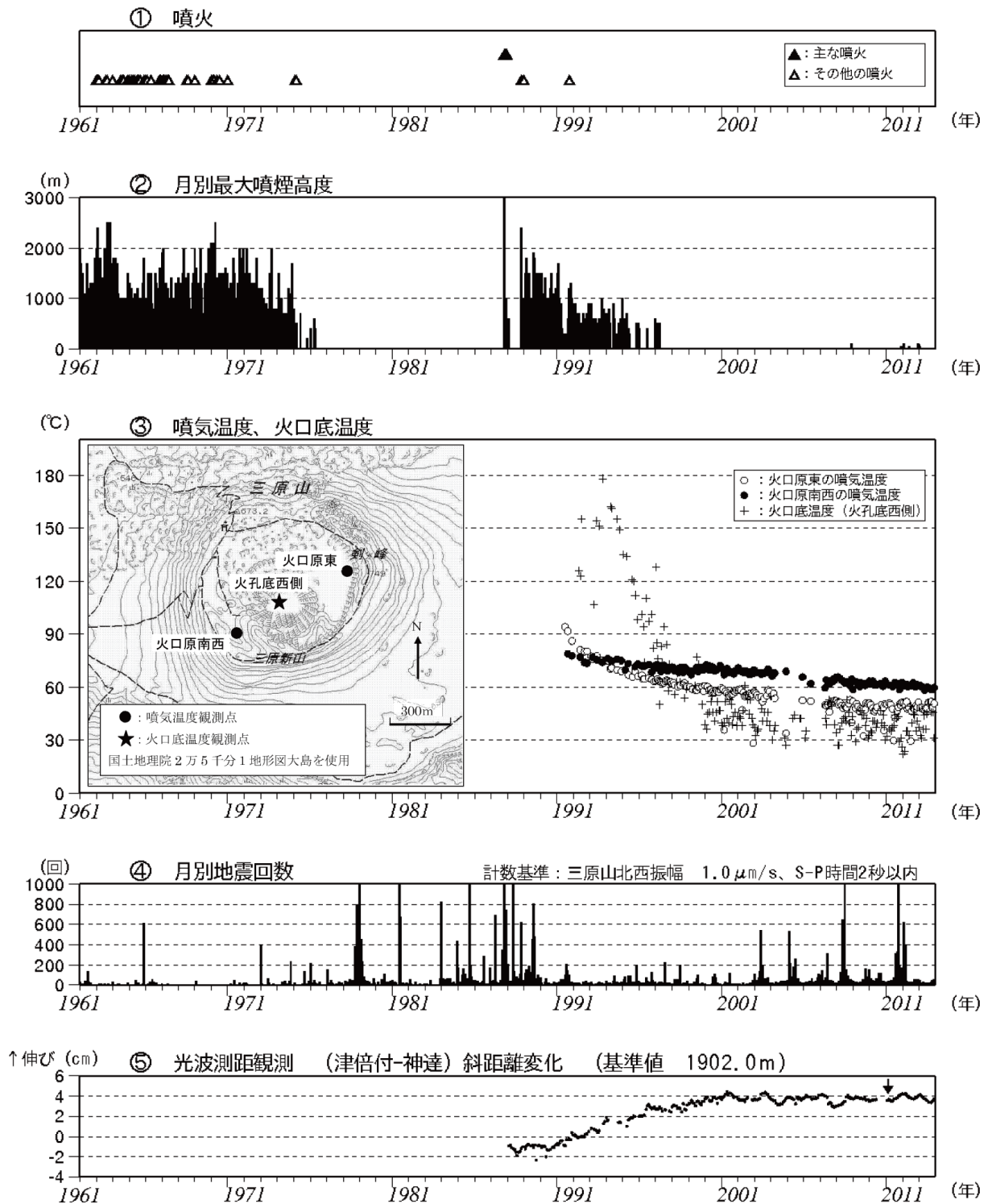
図 1 伊豆大島 長期間の火山活動経過図 (1961 年 1 月～2012 年 12 月)
