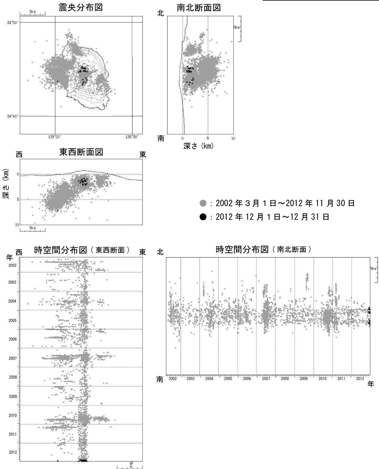
図 7※ 伊豆大島 震源分布図 (2002 年 3 月 1 日 ~ 2012 年 12 月 31 日)
