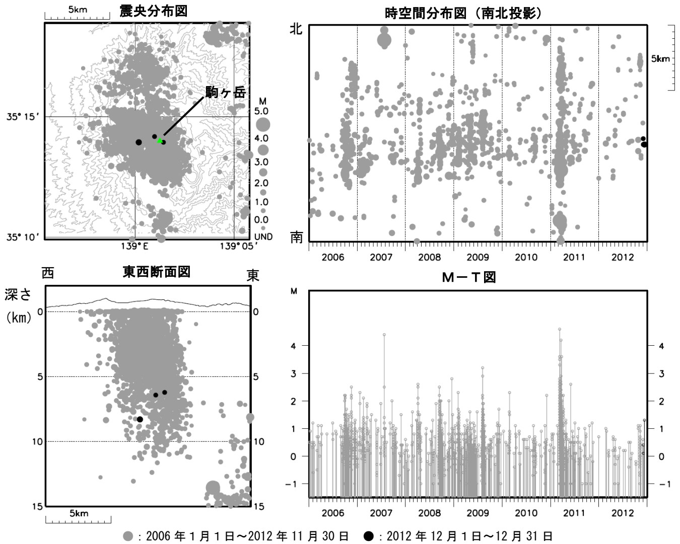
図 4※ 箱根山 広域地震観測網による山体・周辺の震源分布図（2006 年 1 月 1 日～2012 年 12 月 31 日） M（マグニチュード）は地震の規模を表します。 今期間、震源が決定された地震は少なく、地震活動は静穏に経過しました。 図中の震源要素は一部暫定値が含まれており、後日変更することがあります。
