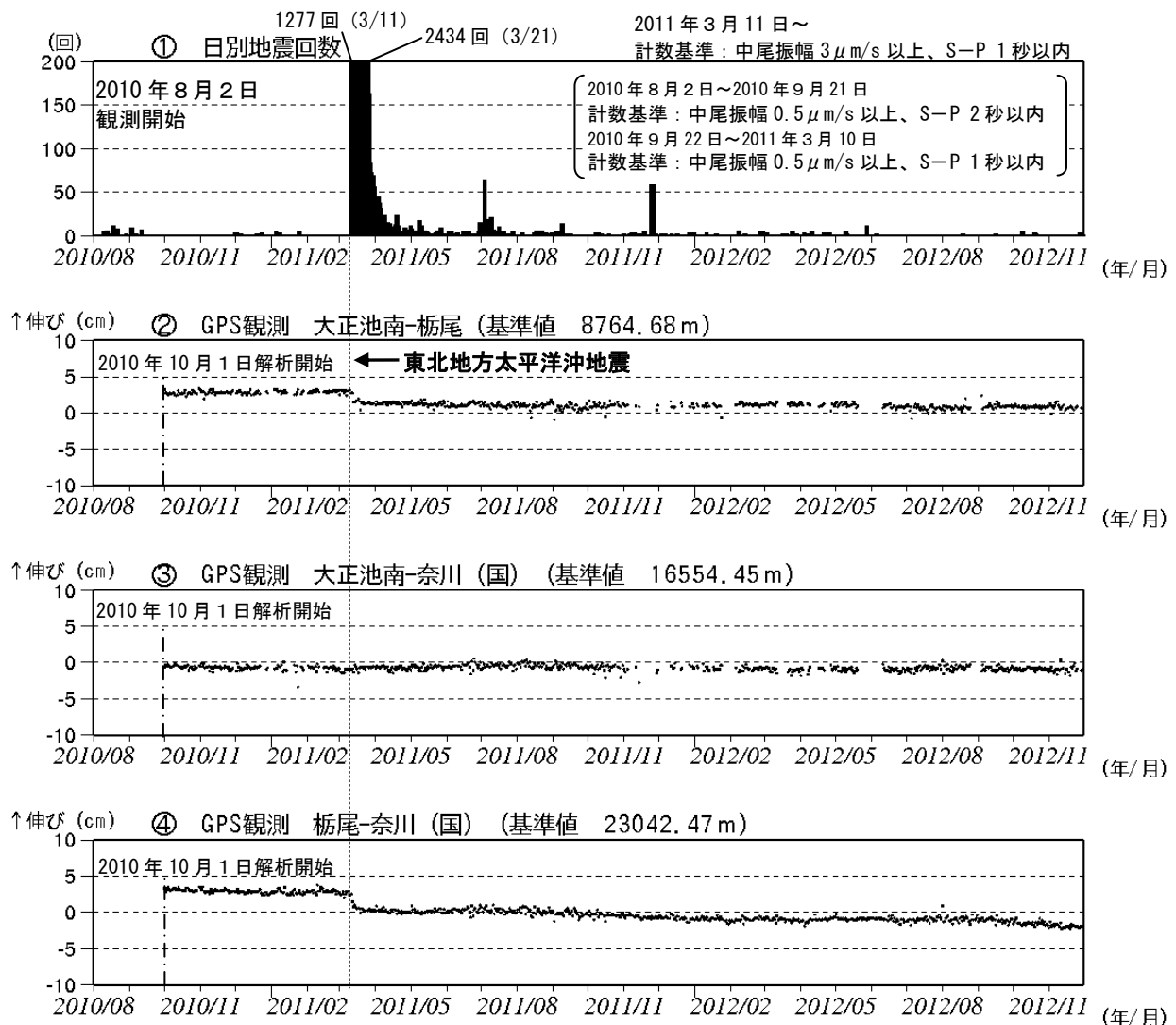
図 3 焼岳 火山活動経過図 (2010 年 8 月 2 日～2012 年 11 月 30 日)
