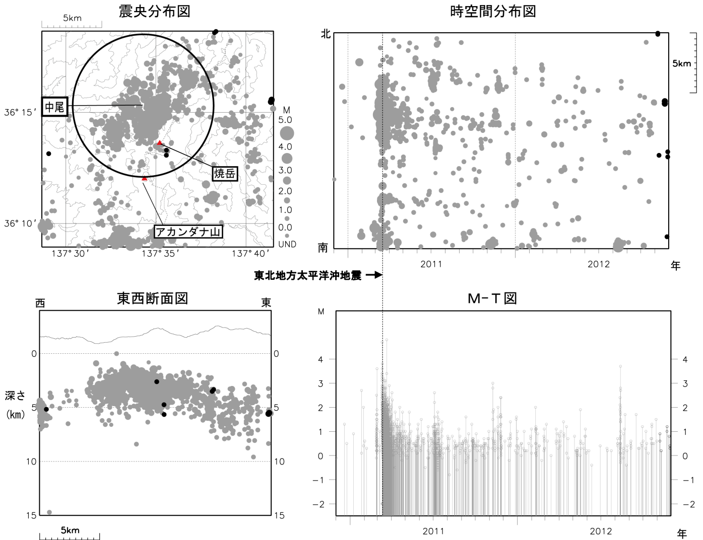
図 4※ 焼岳 広域地震観測網による山体・周辺の地震活動(2010 年 12 月 1 日～2012 年 11 月 30 日)
