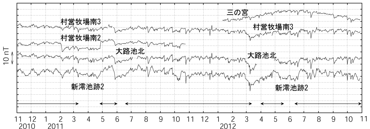
図4 三宅島 全磁力連続観測による全磁力値の変化 (2010年11月～2012年10月)
