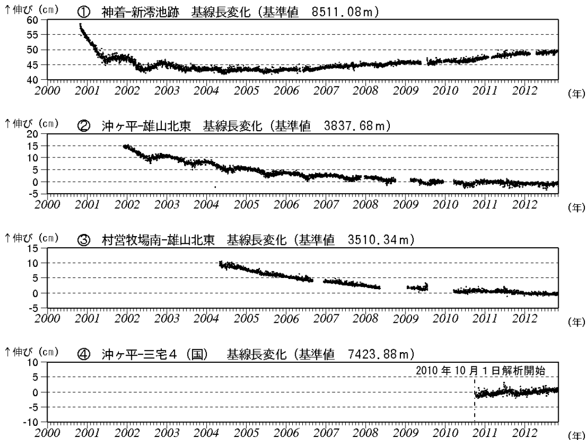
図3 三宅島 GPS 連続観測結果 (2000年1月～2012年10月) (国): 国土地理院 基線①～④※は図7 (観測点配置図) の①～④にそれぞれ対応します。 グラフの空白部分は欠測を示します。 2010年10月以降のデータについては、電離層の影響を補正する等、解析方法を改良しています。
