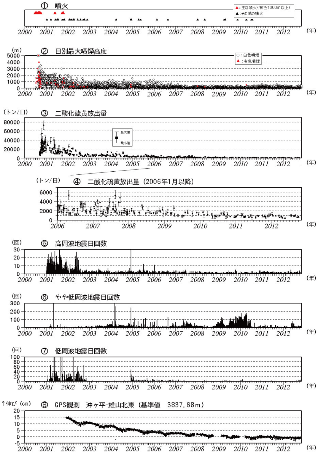
図 2 三宅島 最近の火山活動の経過図 (2000 年 1 月～2012 年 10 月)
