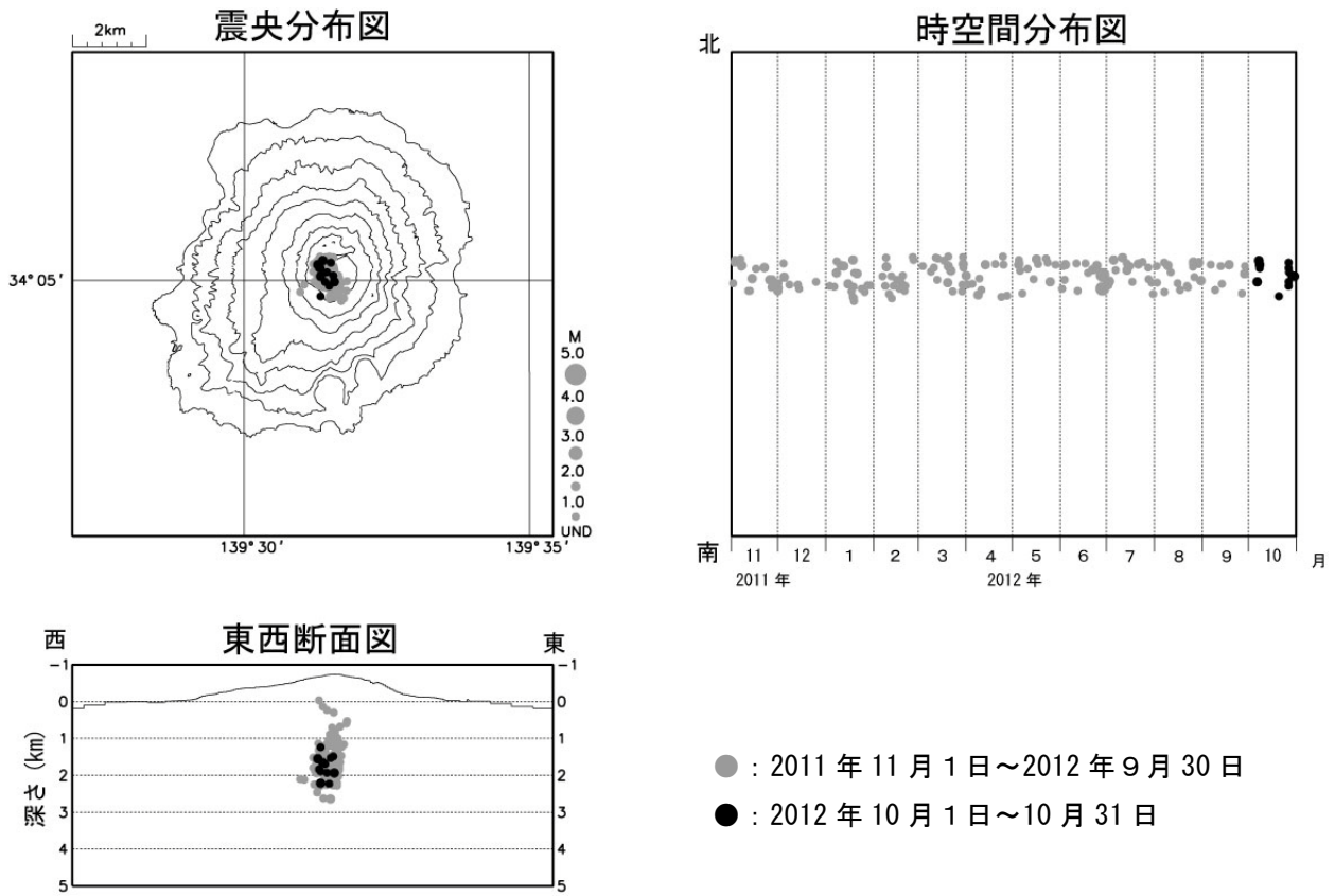
図 5 ※ 三宅島 震源分布図 (2011 年 11 月 1 日 ~ 2012 年 10 月 31 日)
