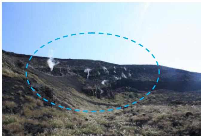
山頂部 (10月19日、北西外輪遠望カメラによる) 剣ガ峰付近 (10月16日、撮影方向は図6参照) 図4 伊豆大島 三原山山頂部及び山頂火口の状況 点円内: ごく弱い噴気
