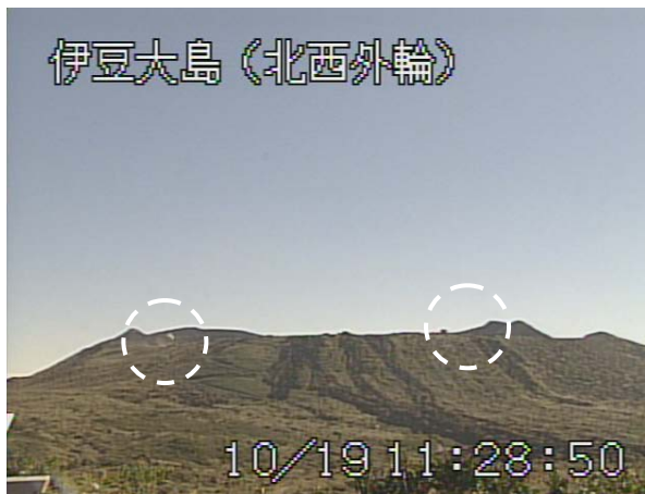
山頂部 (10月19日、北西外輪遠望カメラによる) 剣ガ峰付近 (10月16日、撮影方向は図6参照) 図4 伊豆大島 三原山山頂部及び山頂火口の状況 点円内: ごく弱い噴気
