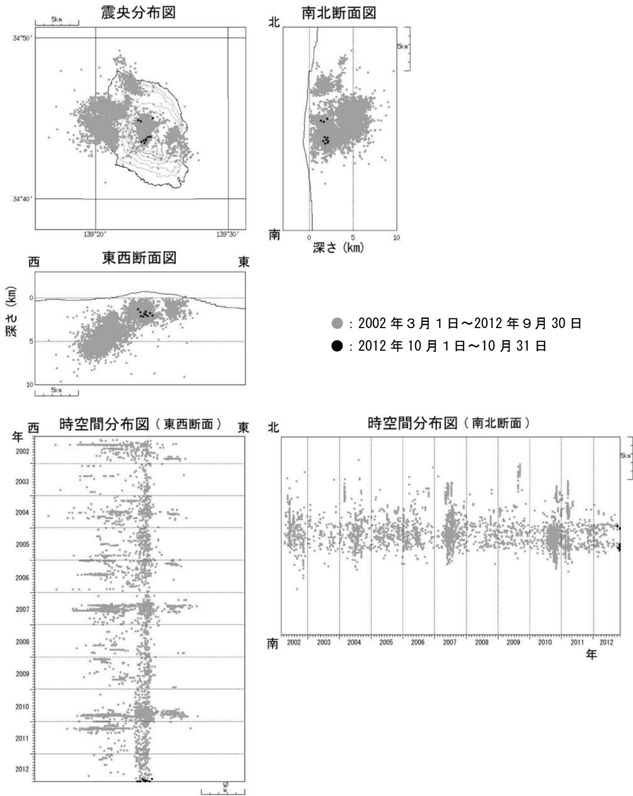
図 7※ 伊豆大島 震源分布図 (2002 年 3 月 1 日 ~ 2012 年 10 月 31 日)
