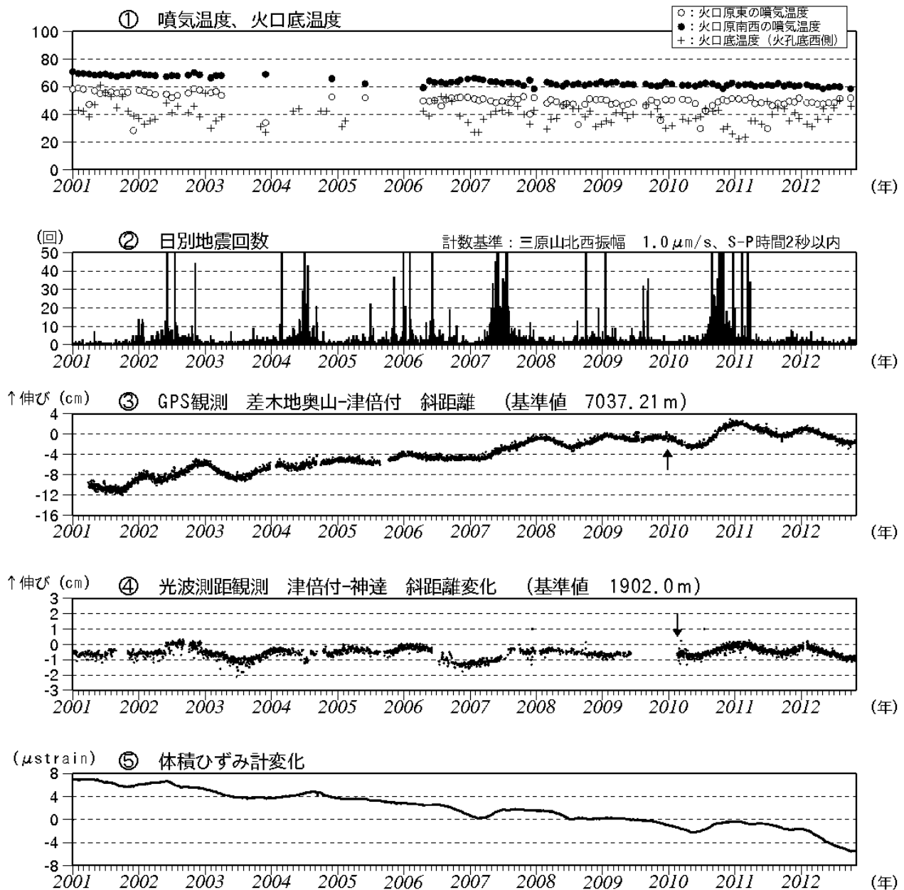
図2 伊豆大島 最近の火山活動経過図 (2001年1月～2012年10月)
