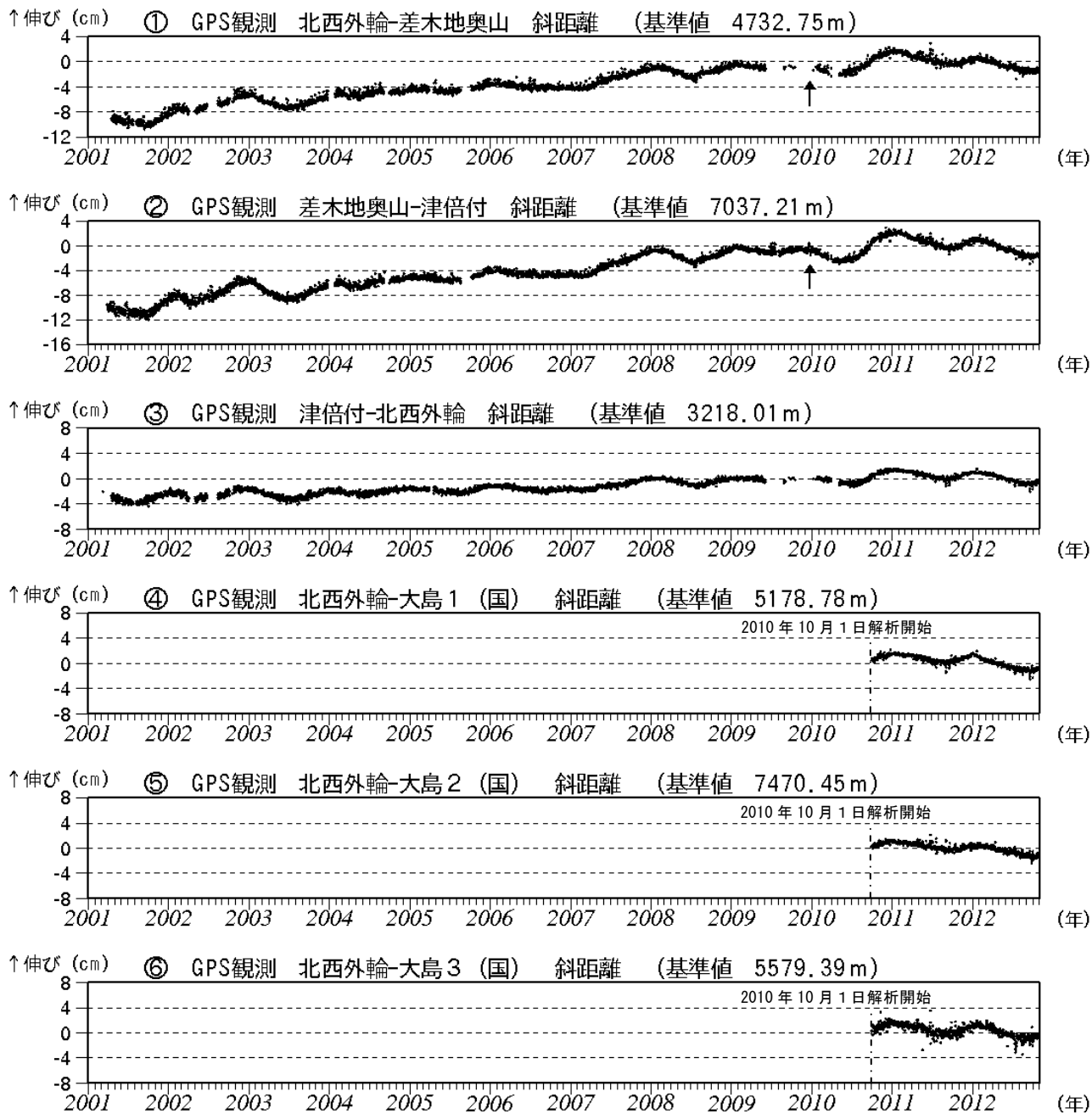
図3※ 伊豆大島 GPS連続観測による基線長変化 (2001年1月~2012年10月) (国): 国土地理院 2010年10月以降のデータについては、電離層の影響を補正する等、解析方法を改良しています。 ①~③、及び④*~⑥*は図8のGPS基線①~⑥に対応しています。 グラフの空白部分は欠測。①②の矢印は差木地奥山支柱工事による変動。
