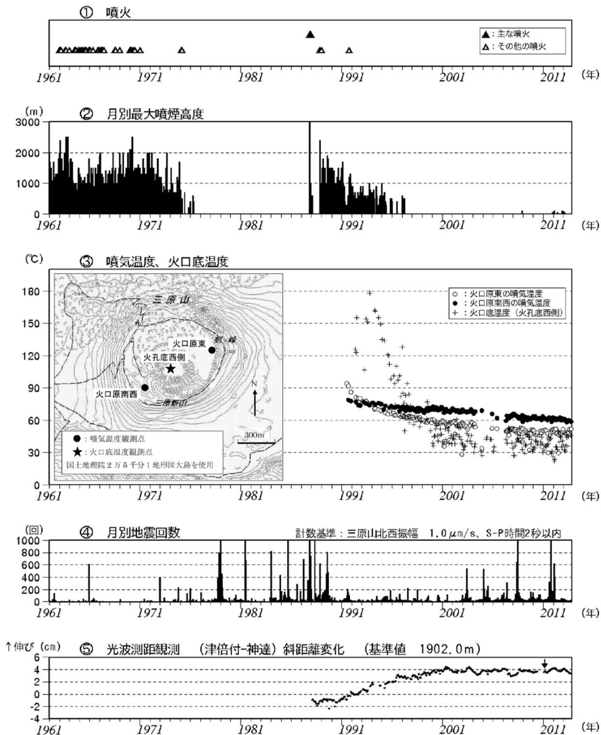
図 1 伊豆大島 長期間の火山活動経過図 (1961 年 1 月~2012 年 10 月)
