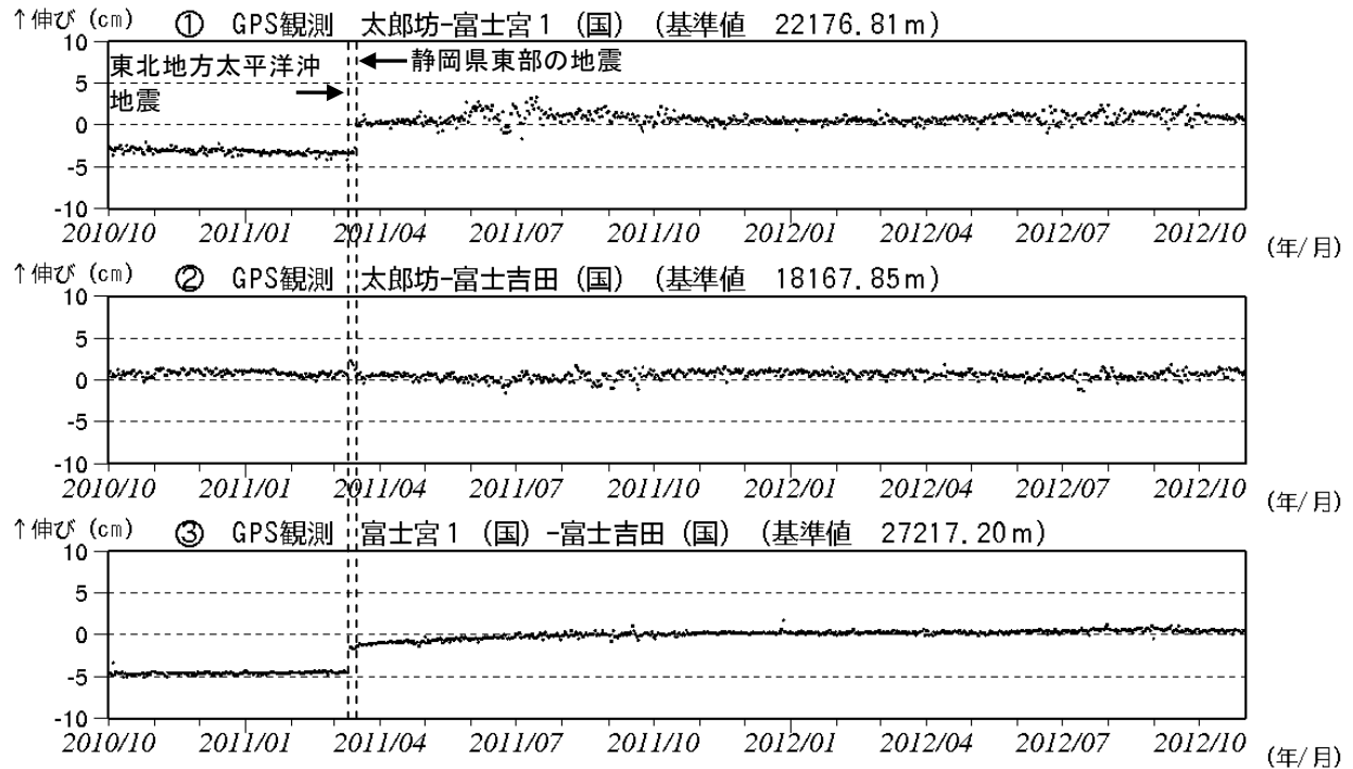
図 4 ※ 富士山 GPS 連続観測による基線長変化（2010 年 10 月 1 日～2012 年 10 月 31 日） （国）：国土地理院
