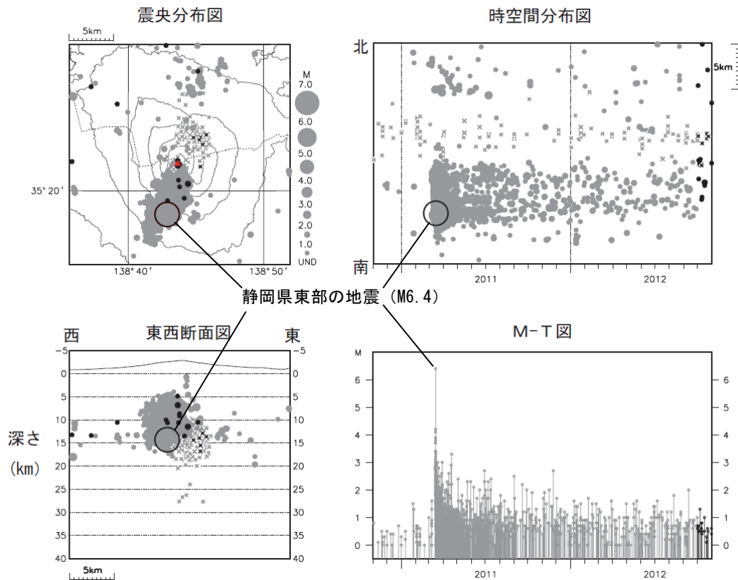
図 3 ※ 富士山 広域地震観測網による山体・周辺の地震活動（2010 年 11 月 1 日～2012 年 10 月 31 日）
