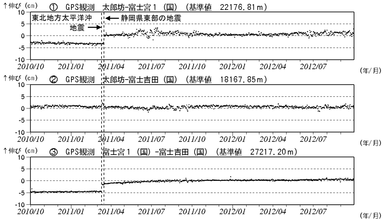
図 4 ※ 富士山 GPS 連続観測による基線長変化（2010 年 10 月 1 日～2012 年 9 月 30 日） （国）：国土地理院
