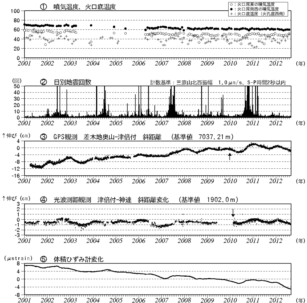
図2 伊豆大島 最近の火山活動経過図（2001年1月～2012年8月）
