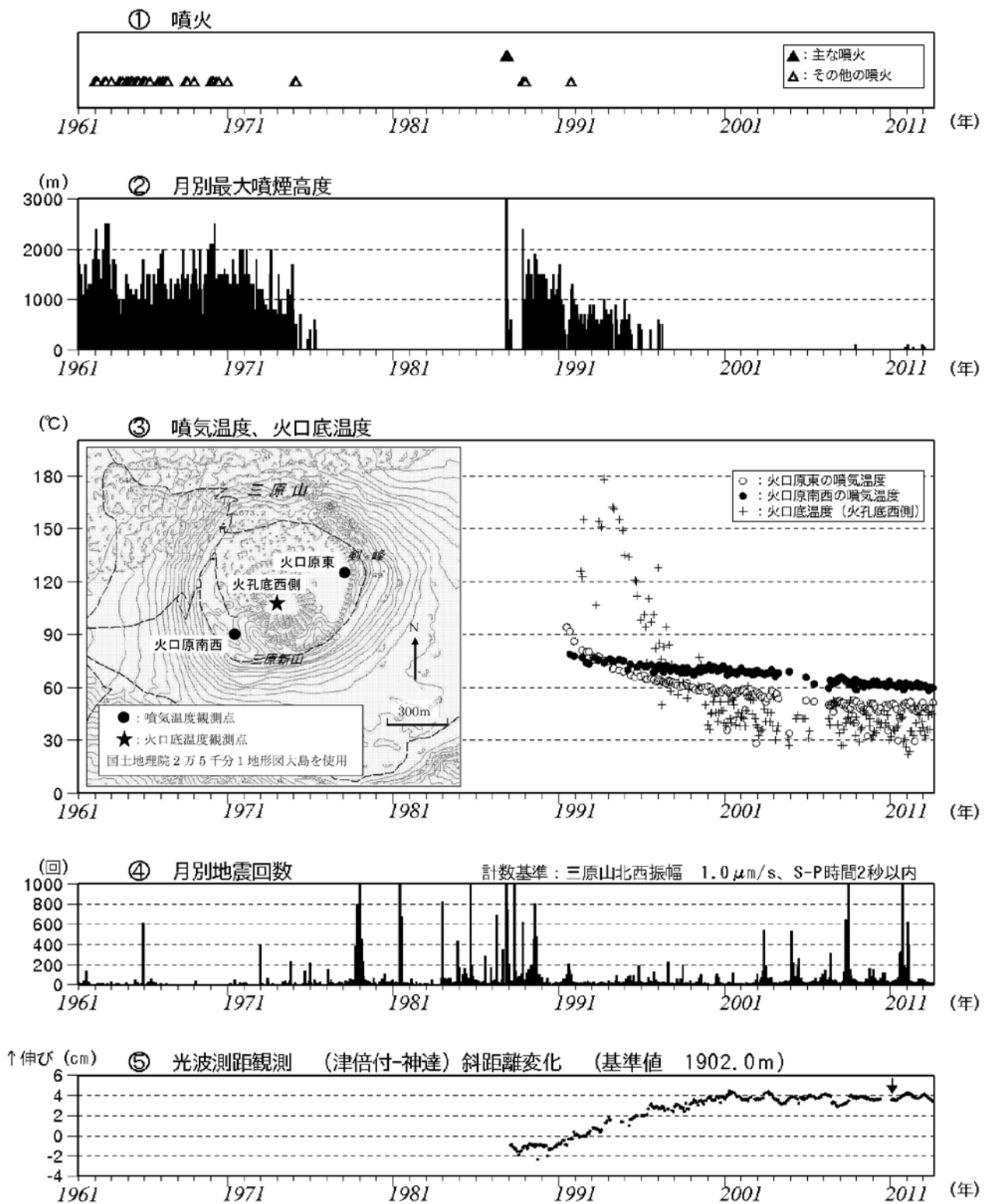
図 1 伊豆大島 長期間の火山活動経過図（1961 年 1 月～2012 年 8 月）
