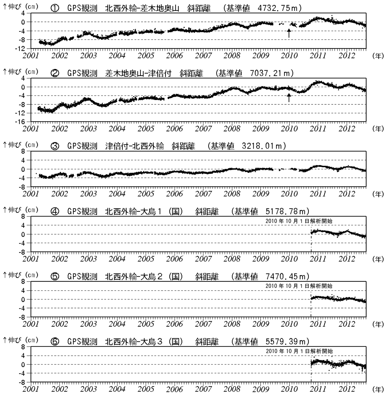
図3※ 伊豆大島 GPS連続観測による基線長変化（2001年1月～2012年8月）（国）：国土地理院 2010年10月以降のデータについては、電離層の影響を補正する等、解析方法を改良しています。 ①～③、及び④※～⑥※は図8のGPS基線①～⑥に対応しています。 グラフの空白部分は欠測。①②の矢印は差木地奥山支柱工事による変動。
