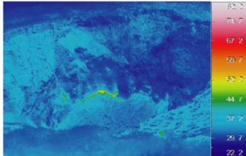
図5 伊豆大島 中央火孔内の状況（左）と地表面温度分布 1) （右）
