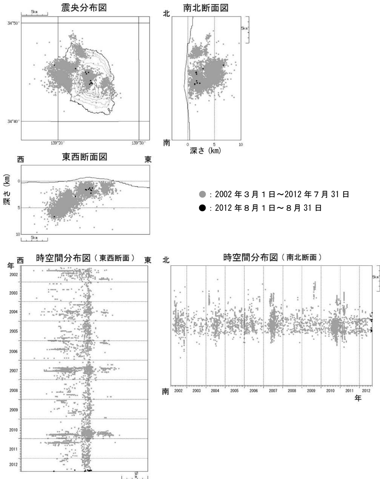
図 7※ 伊豆大島 震源分布図 (2002 年 3 月 1 日 ~ 2012 年 8 月 31 日)
