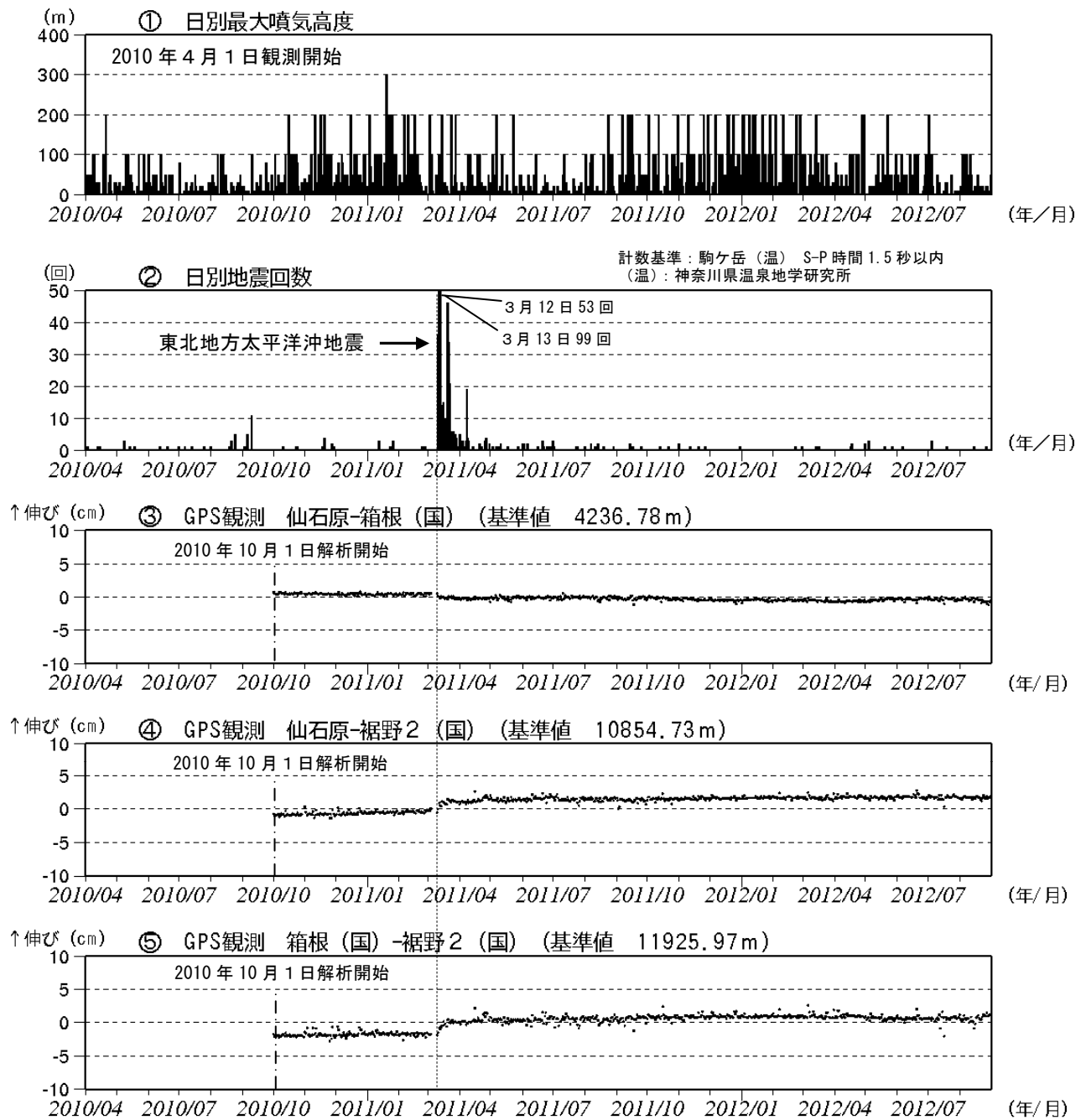
図 3 箱根山 火山活動経過図（2010 年 4 月 1 日～2012 年 8 月 31 日）
