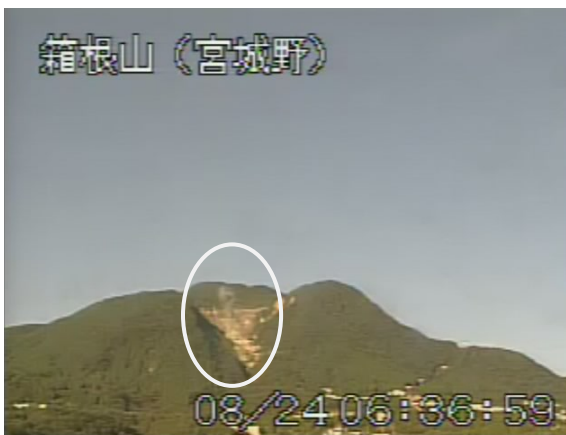
図 1 箱根山 早雲地獄の状況 （8 月 24 日、宮城野遠望カメラによる） 白円内は早雲地獄からの噴気。
