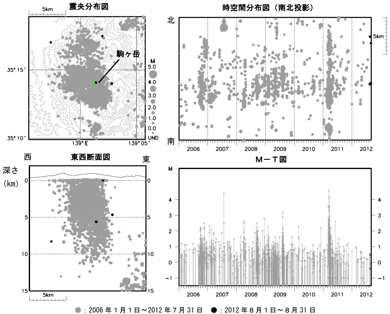
図 4 ※ 箱根山 広域地震観測網による山体・周辺の震源分布図（2006 年 1 月 1 日～2012 年 8 月 31 日） M（マグニチュード）は地震の規模を表します。 今期間、震源が決定された地震は少なく、地震活動は静穏に経過しました。 図中の震源要素は一部暫定値が含まれており、後日変更することがあります。
