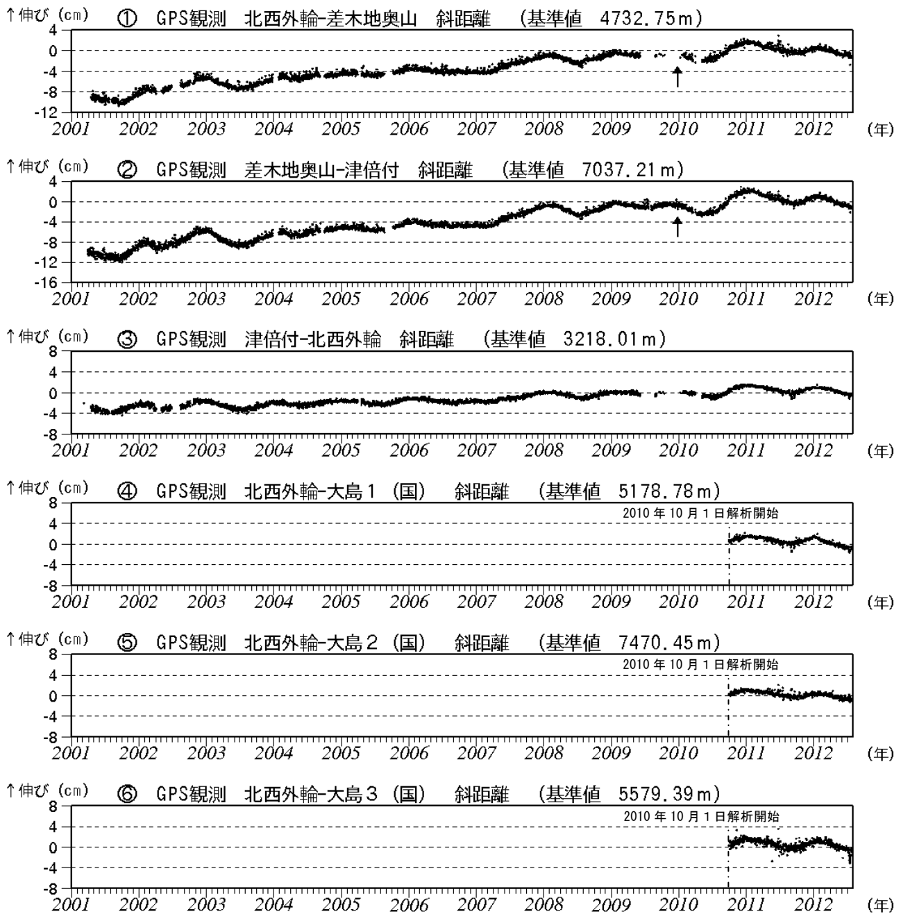
図3※ 伊豆大島 GPS連続観測による基線長変化 (2001年1月~2012年7月) (国): 国土地理院 2010年10月以降のデータについては、電離層の影響を補正する等、解析方法を改良しています。 ①~③、及び④*~⑥*は図8のGPS基線①~⑥に対応しています。 グラフの空白部分は欠測。①②の矢印は差木地奥山支柱工事による変動。
