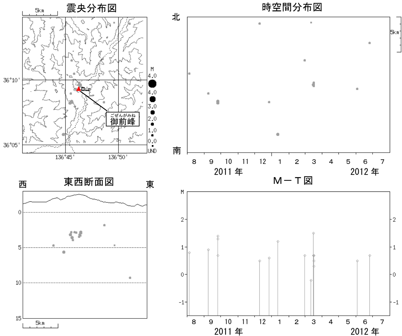
図 4 ※白山 広域地震観測網による山体・周辺の地震活動（2011 年 8 月～2012 年 7 月）
