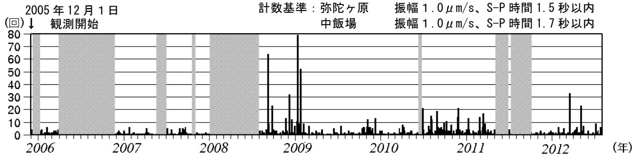
図 3 白山 日別地震回数（2005 年 12 月～2012 年 7 月）
