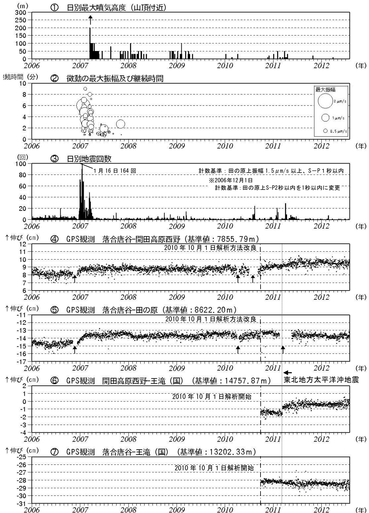
図3 御嶽山 最近の火山活動経過図（2006年1月1日～2012年7月31日）
