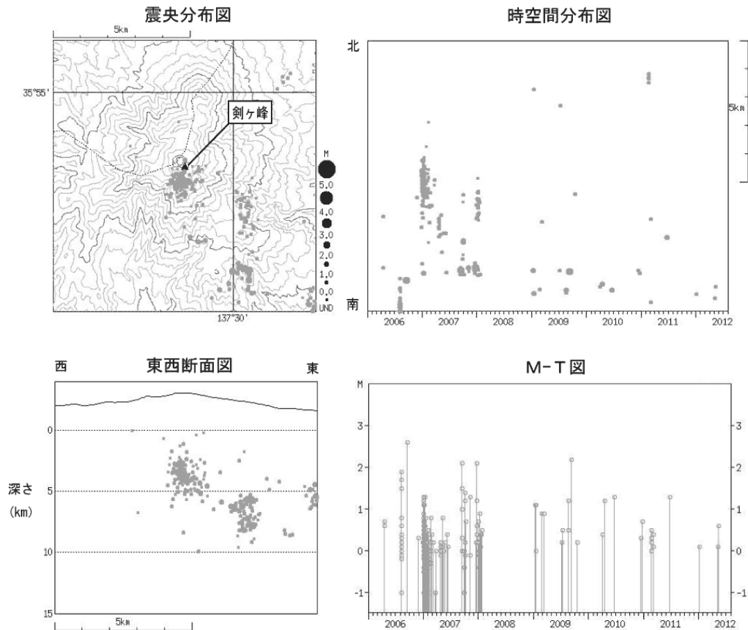
図 4 ※ 御嶽山 広域地震観測網による山体・周辺の震源分布図（2006 年 1 月 1 日～2012 年 7 月 31 日） ●：2006 年 1 月 1 日～2012 年 6 月 30 日 ●：2012 年 7 月 1 日～7 月 31 日 M（マグニチュード）は地震の規模を表します。 今期間、震源が決定された地震はありません。 図中の震源要素は一部暫定値が含まれており、後日変更することがあります。
