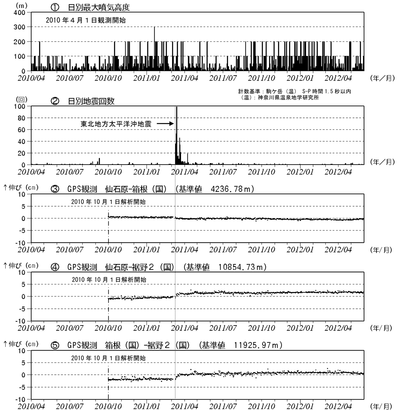
図3 箱根山 火山活動経過図（2010年4月1日～2012年5月31日）
