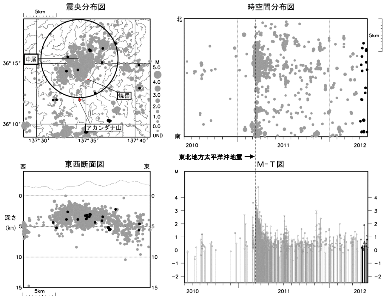
図 4※ 焼岳 広域地震観測網による山体・周辺の地震活動（2010 年 6 月 1 日～2012 年 5 月 31 日）
