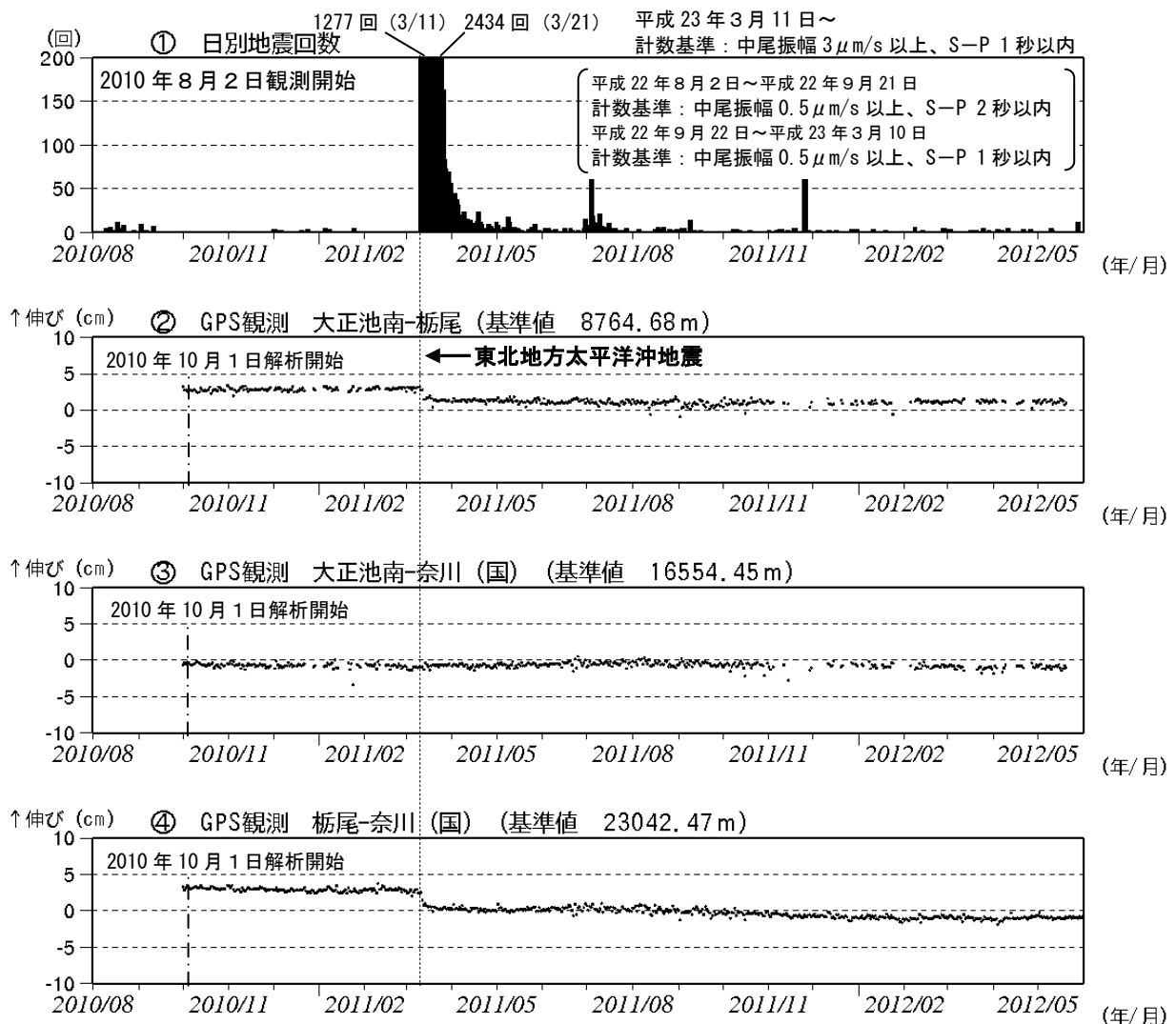
図 3 焼岳 火山活動経過図（2010年 8 月 2 日～2012年 5 月31日）
