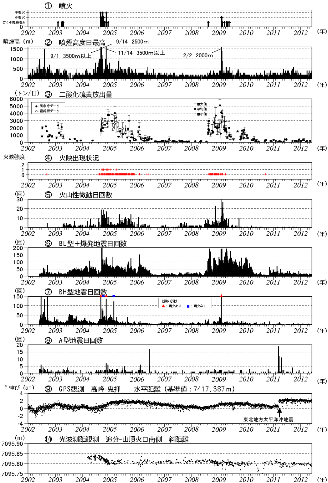
図 5※ 浅間山 最近の火山活動経過図（2002 年 1 月 1 日～2012 年 5 月 31 日）
