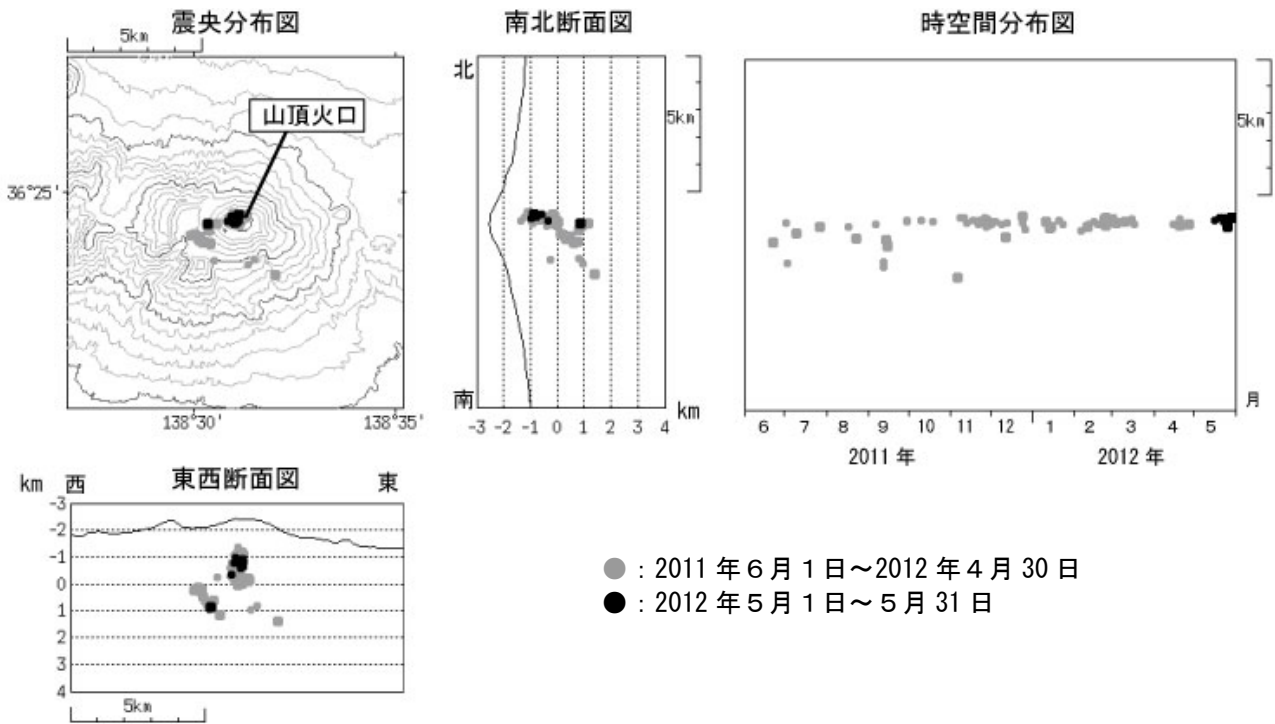
図 6※ 浅間山 震源分布図 (2011 年 6 月 1 日～2012 年 5 月 31 日)
