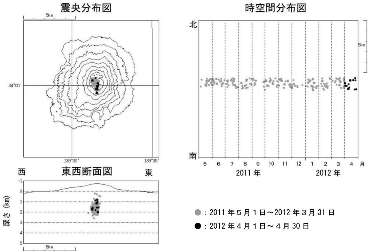
図 5※ 三宅島 震源分布図 (2011 年 5 月 1 日~2012 年 4 月 30 日)
