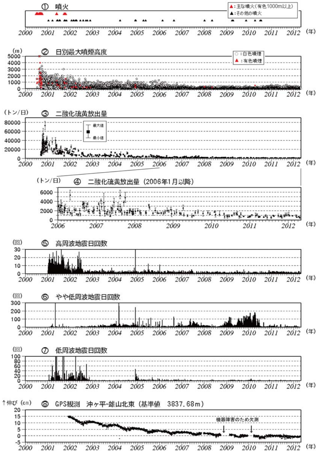
図2 三宅島 最近の火山活動の経過図（2000年1月～2012年4月）
