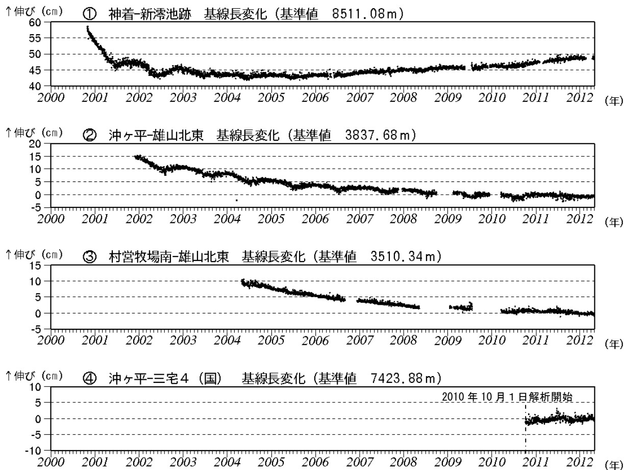
図3 三宅島 GPS 連続観測結果（2000年1月～2012年4月）（国）：国土地理院 基線①～④※は図7（観測点配置図）の①～④にそれぞれ対応します。 グラフの空白部分は欠測を示します。 2010年10月以降のデータについては、電離層の影響を補正する等、解析方法を改良しています。
