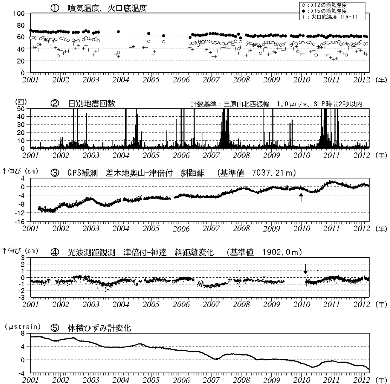
図2 伊豆大島 最近の火山活動経過図（2001年1月～2012年3月）
