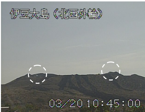
山頂部（3月20日、北西外輪遠望カメラによる） 剣ガ峰付近（3月21日、撮影方向は図6参照） 図4 伊豆大島 三原山山頂火口内及び山頂部の状況 点円内：ごく弱い噴気
