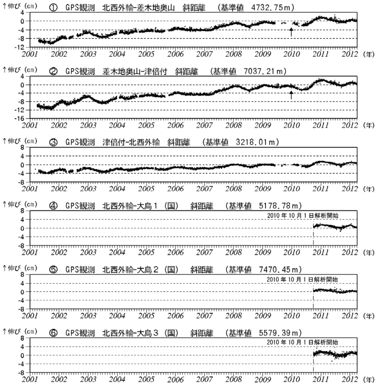
図3※ 伊豆大島 GPS連続観測による基線長変化 (2001年1月~2012年3月) (国): 国土地理院 2010年10月以降のデータについては、電離層の影響を補正する等、解析方法を改良しています。 ①~③、及び④※~⑥※は図8のGPS基線①~⑥に対応しています。 グラフの空白部分は欠測。①②の矢印は差木地奥山支柱工事による変動。
