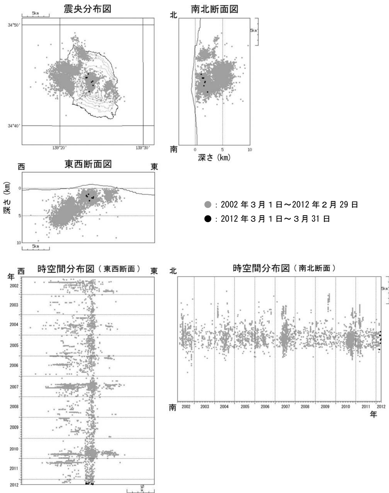
図 7 ※ 伊豆大島 震源分布図 (2002 年 3 月 1 日～2012 年 3 月 31 日)
