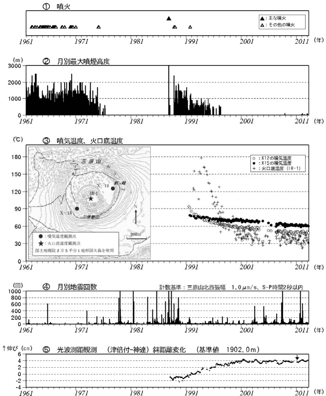
図 1 伊豆大島 長期間の火山活動経過図（1961 年 1 月～2012 年 3 月）
