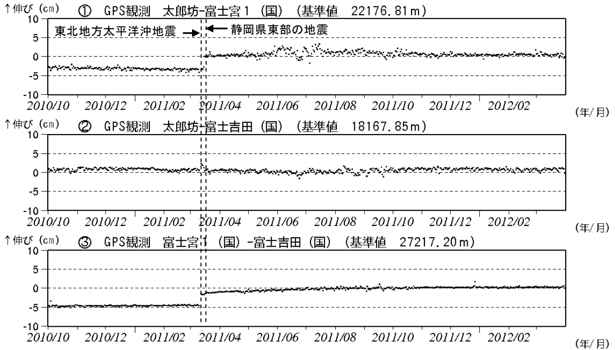
図 4 * 富士山 GPS 連続観測による基線長変化 (2010 年 10 月 1 日~2012 年 3 月 31 日) (国): 国土地理院
