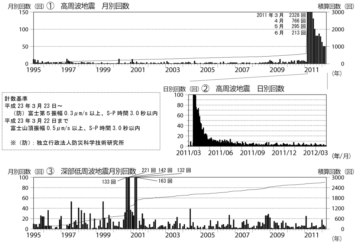
図 2 ※ 富士山 月別及び日別地震回数（1995 年 6 月～2012 年 3 月）
