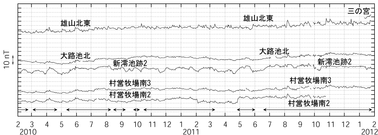
図 4 三宅島 全磁力連続観測による全磁力値の変化（2010 年 2 月～2012 年 1 月）
