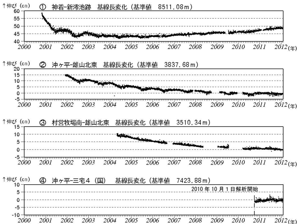
図 3 三宅島 GPS 連続観測結果（2000 年～2012 年 1 月）（国）：国土地理院
