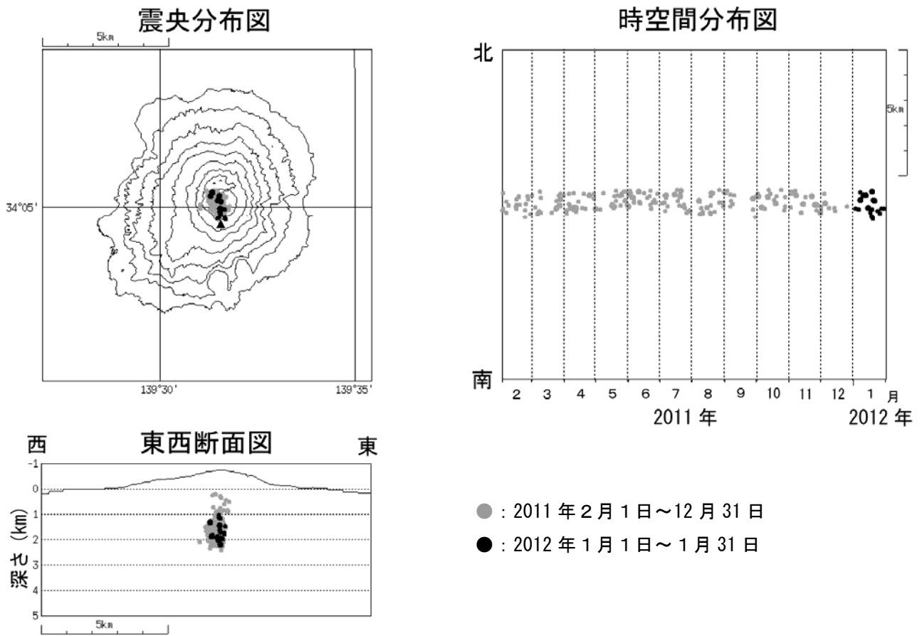
図 5※ 三宅島 震源分布図 (2011 年 2 月 1 日 ~ 2012 年 1 月 31 日)
