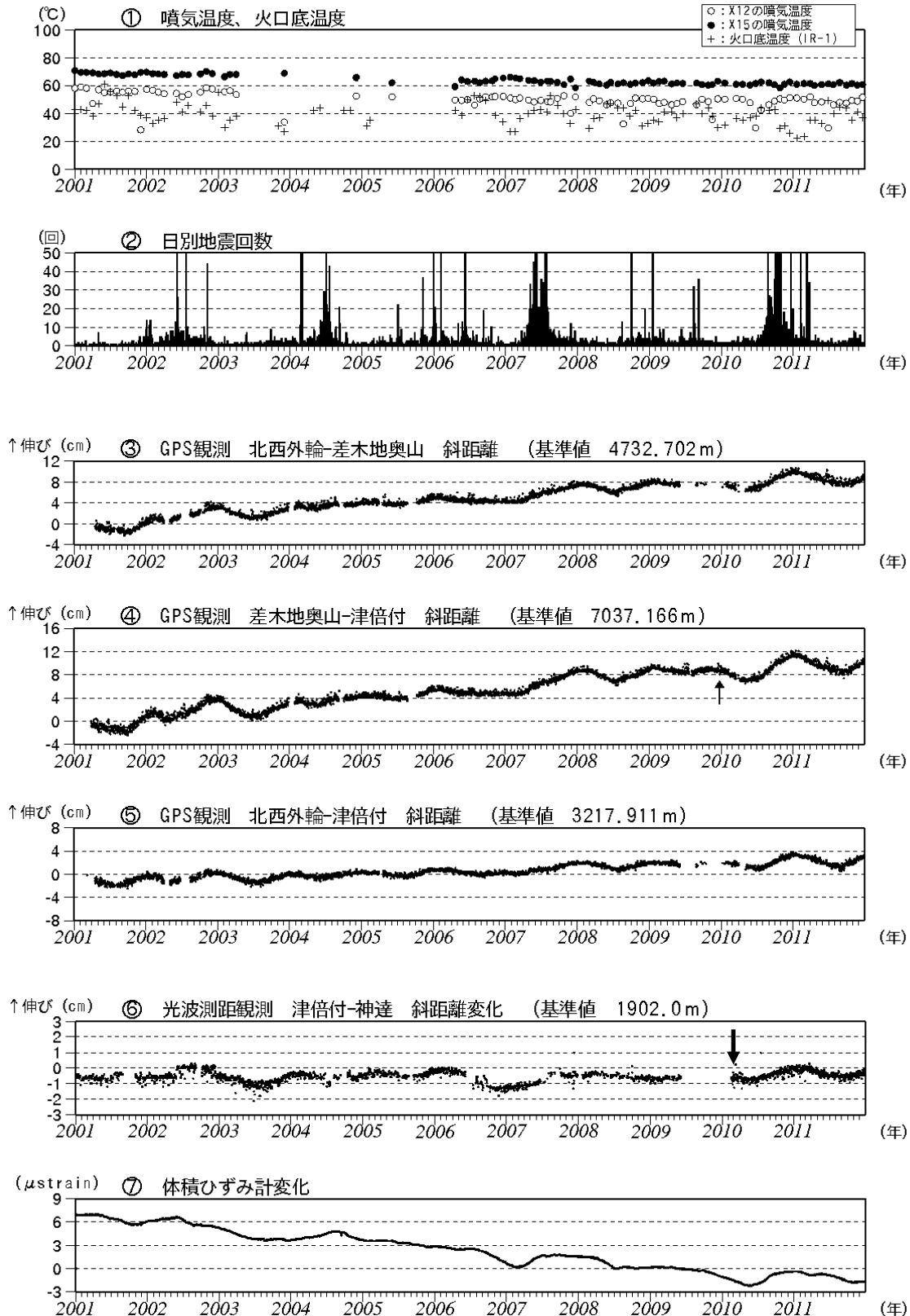
図2 伊豆大島 最近の火山活動経過図 (2001年1月～2011年12月)
