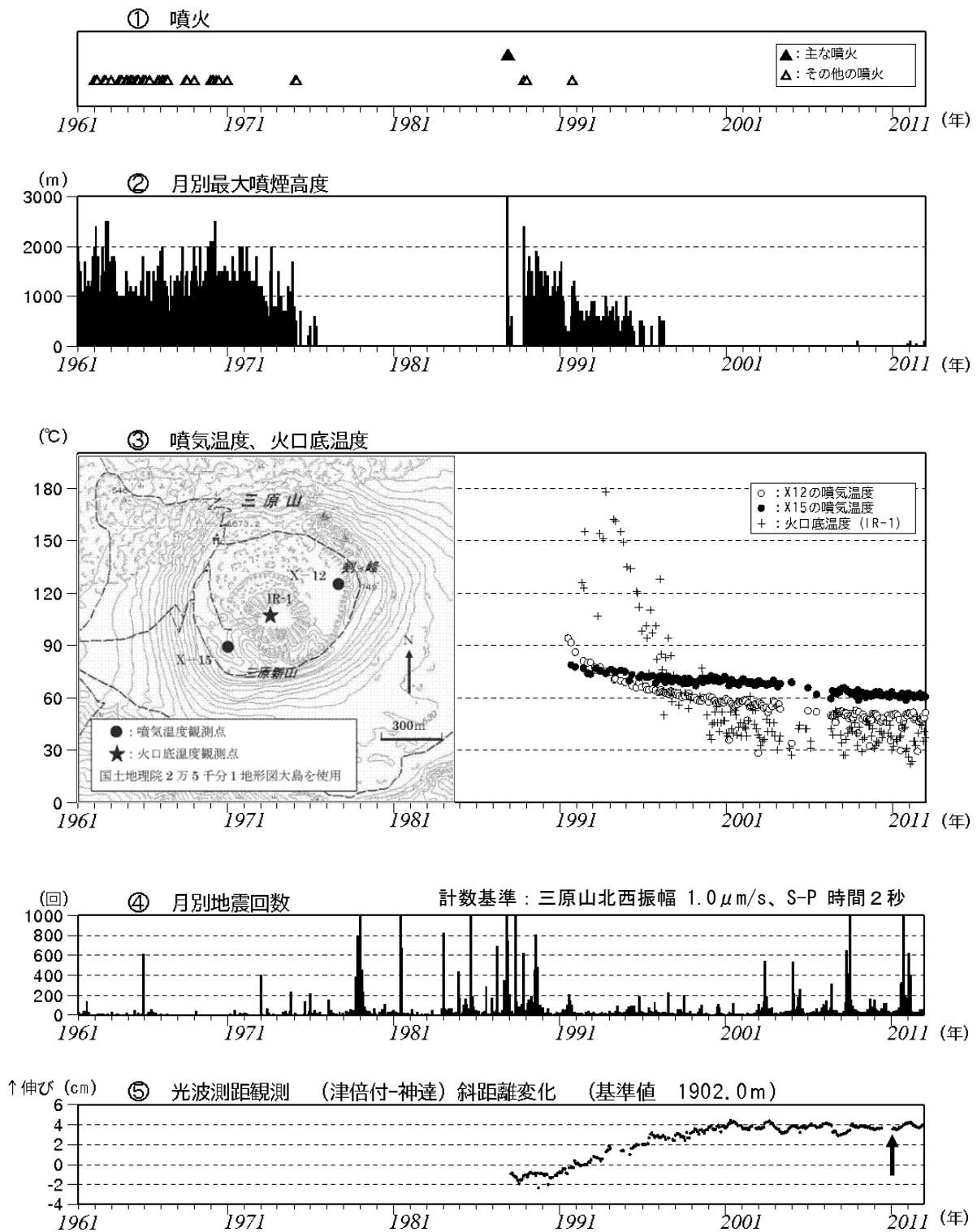
図 1 伊豆大島 長期間の火山活動経過図 (1961 年 1 月～2011 年 12 月)
