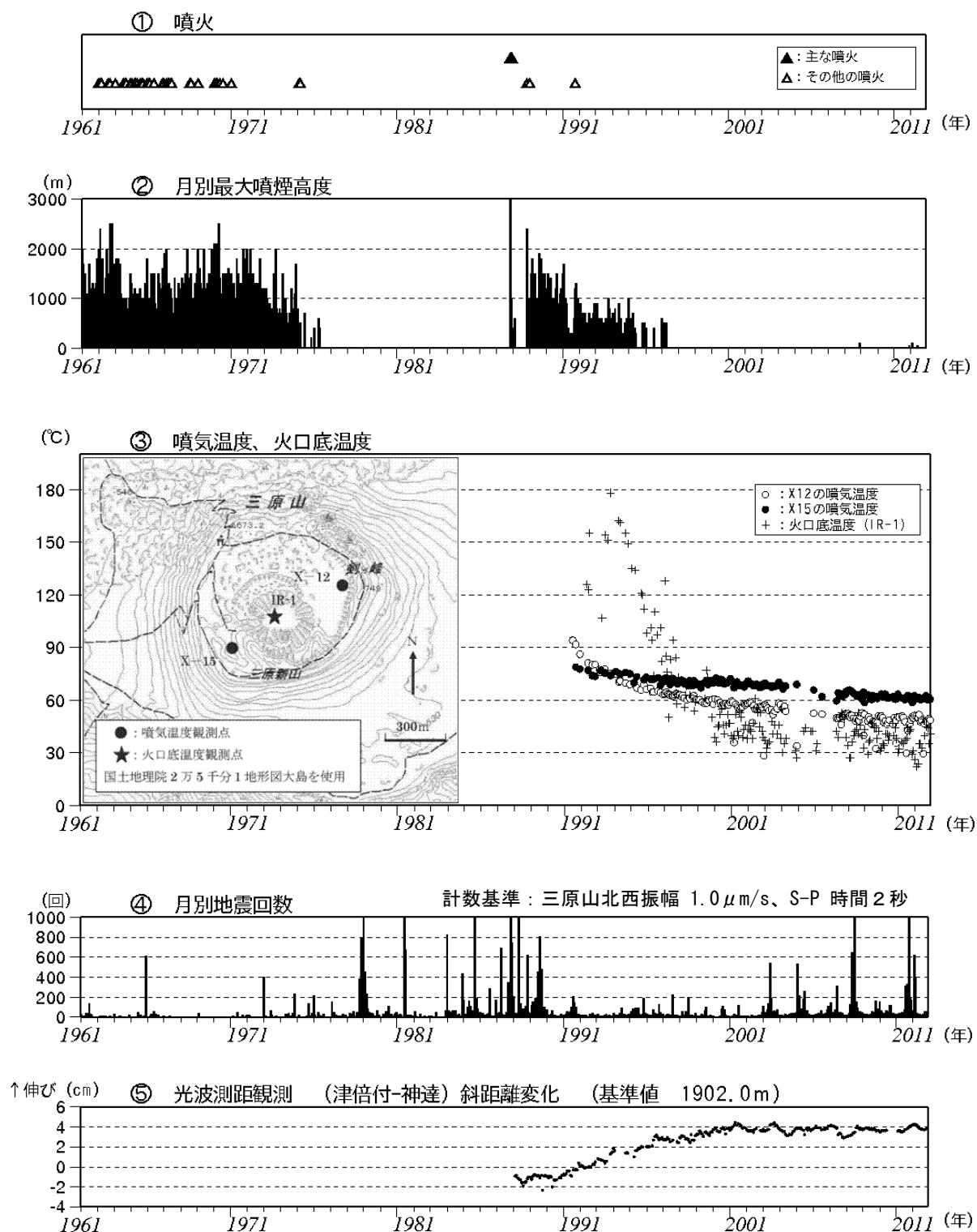
図 1 伊豆大島 長期間の火山活動経過図（1961 年 1 月～2011 年 11 月）
