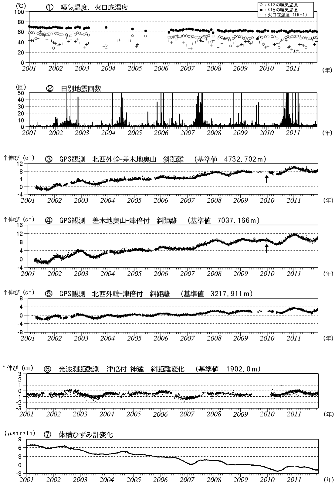
図2 伊豆大島 最近の火山活動経過図（2001年1月～2011年11月）
