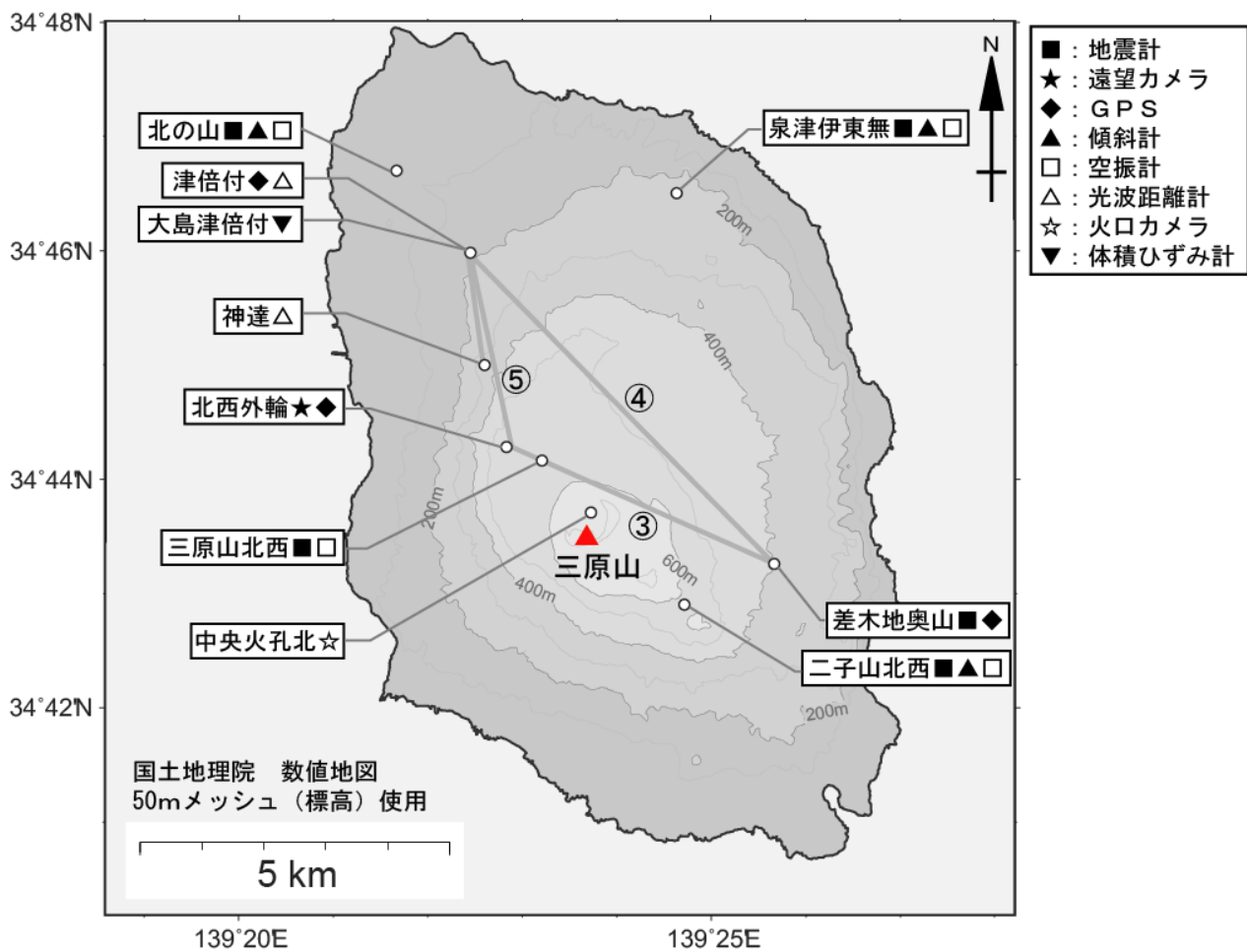
図7 伊豆大島 気象庁の観測点配置図（小さな白丸は観測点位置を示しています） 図中の③～⑤は図2のGPS基線③～⑤に対応しています。
