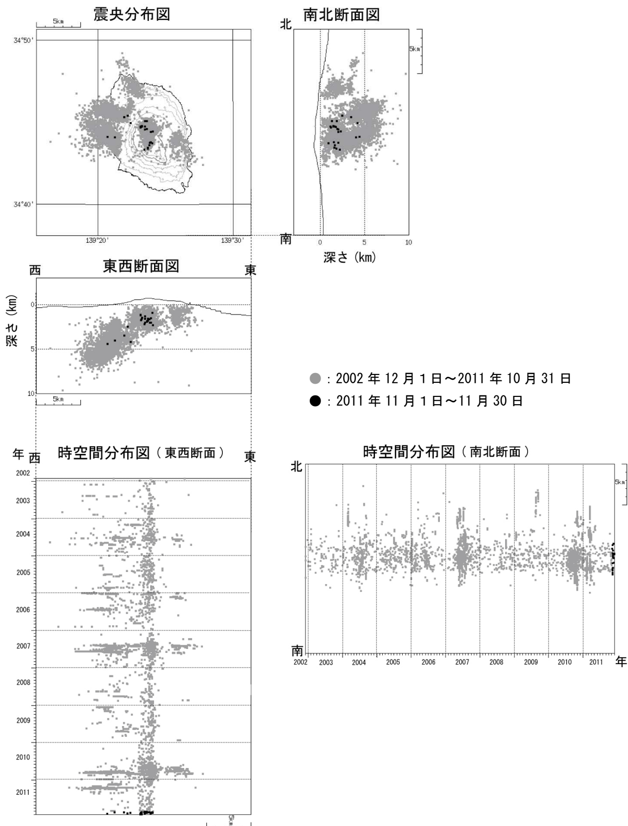
図 6※ 伊豆大島 震源分布図（2002 年 12 月 1 日～2011 年 11 月 30 日）
