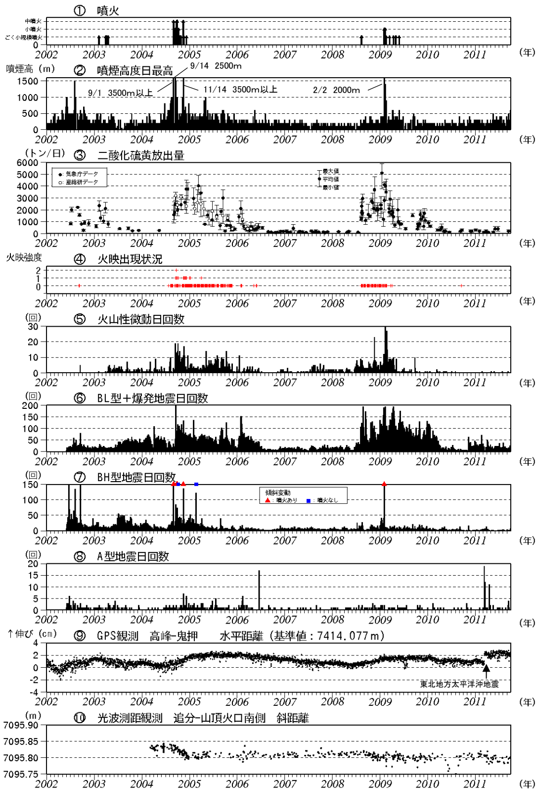
図3※ 浅間山 最近の火山活動の推移（2002年1月1日～2011年9月30日）
