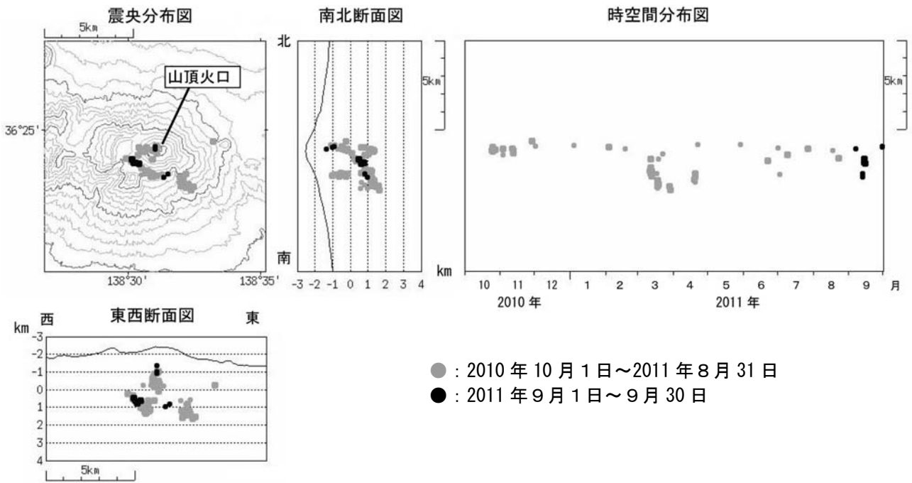
図 4 ※ 浅間山 震源分布図 (2010 年 10 月 1 日～2011 年 9 月 30 日)
