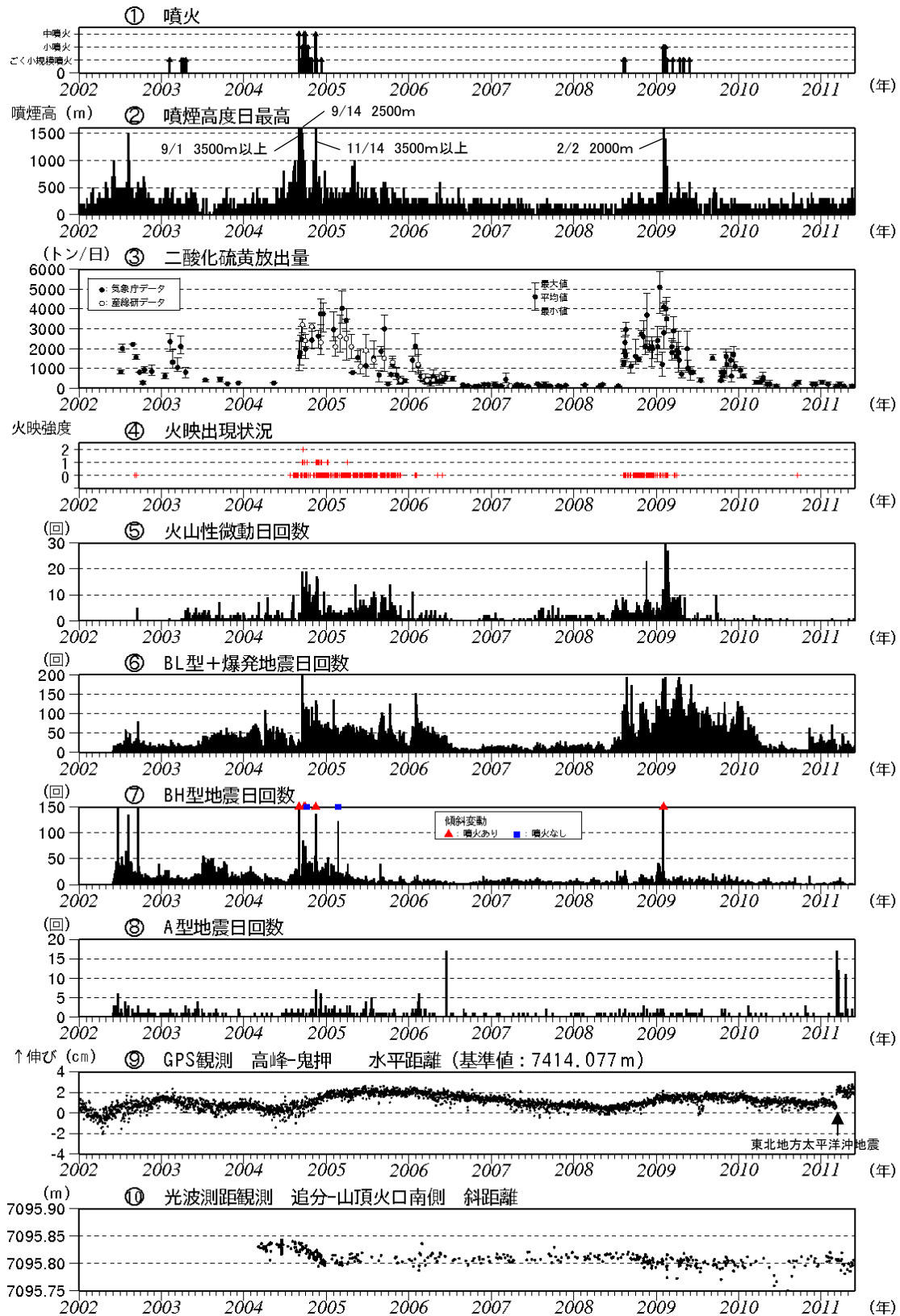
図3※ 浅間山 最近の火山活動の推移（2002年1月1日～2011年5月31日）
