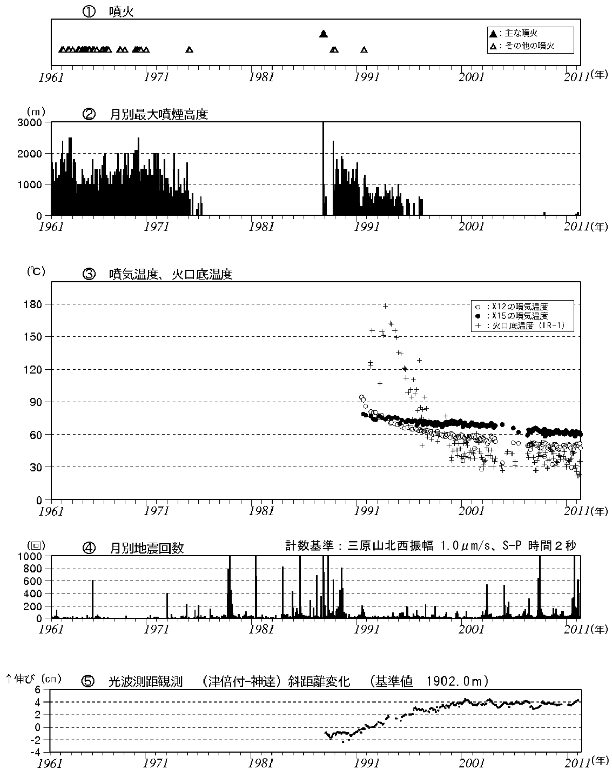
図 1 伊豆大島 長期間の火山活動経過図（1961 年 1 月～2011 年 4 月）
