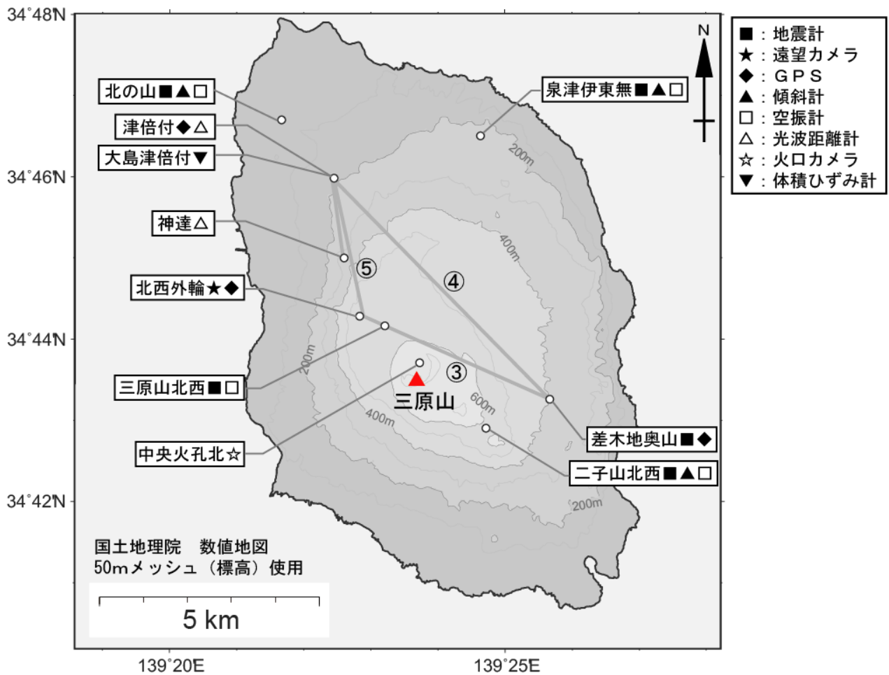
図7 伊豆大島 気象庁の観測点配置図 (小さな白丸は観測点位置を示しています) 図中の③～⑤は図2のGPS基線③～⑤に対応しています。 伊東無、大清水、千波、志久保観測点は3月31日に廃止しました。
