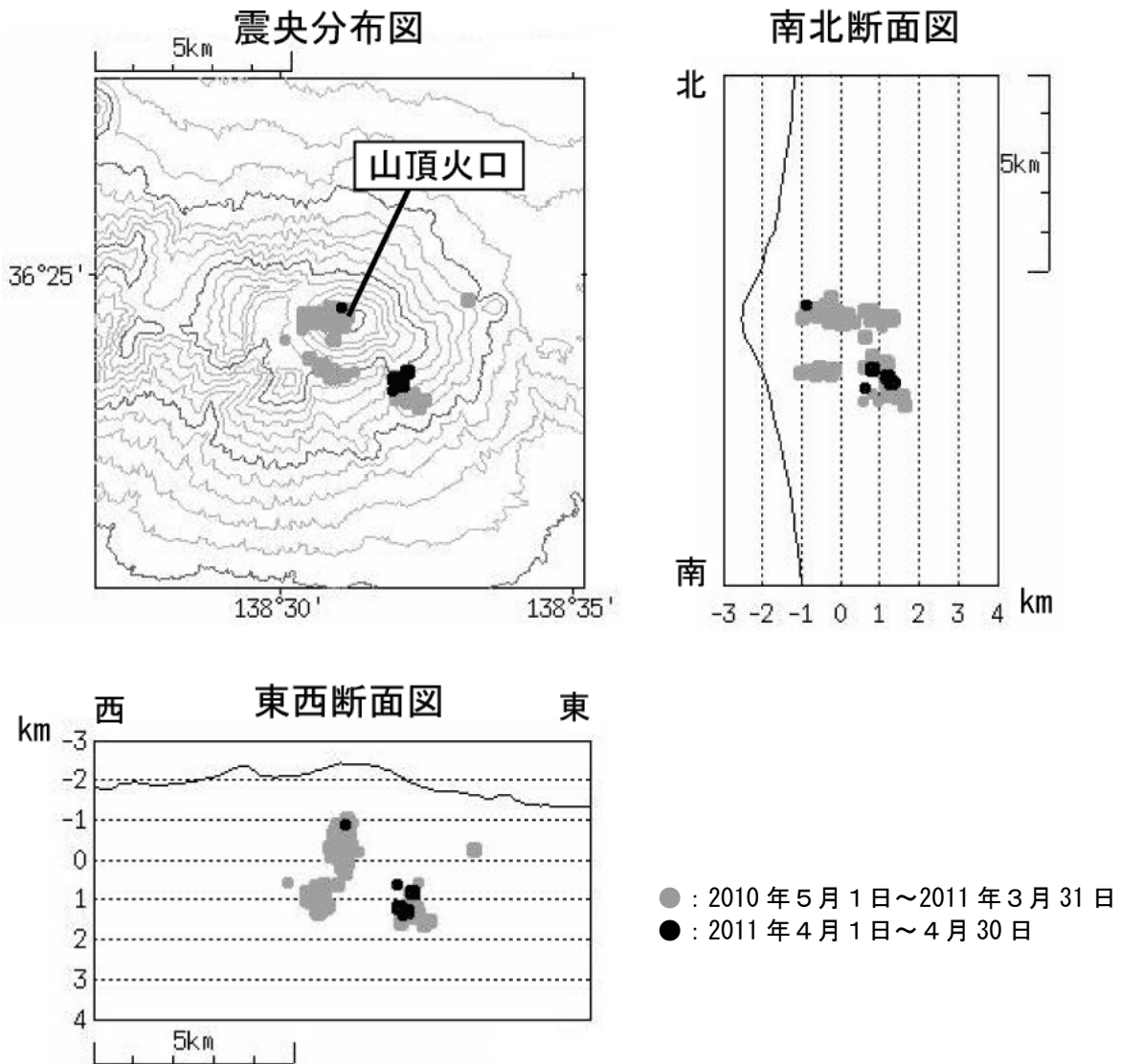
図 4※ 浅間山 震源分布図（2010 年 5 月 1 日～2011 年 4 月 30 日）
