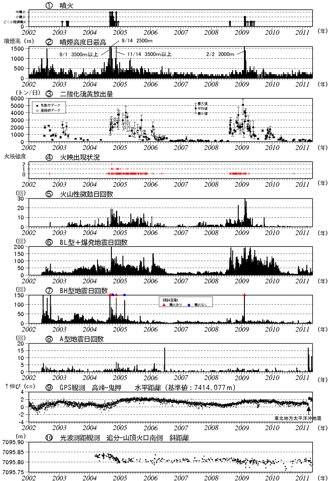
図 3※ 浅間山 最近の火山活動の推移（2002 年 1 月 1 日～2011 年 4 月 30 日）
