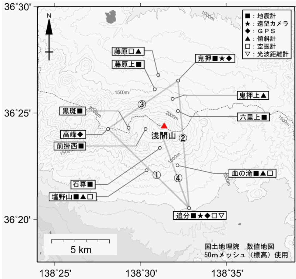
図 1 浅間山 気象庁の観測点配置図（小さな白丸は観測点位置を示しています） GPS 基線③は図 3 の⑨に、光波測距測線④は図 3 の⑩にそれぞれ対応しています。 運用開始前の観測点も含まれます。大窪沢観測点は 3 月 31 日に廃止しました。
