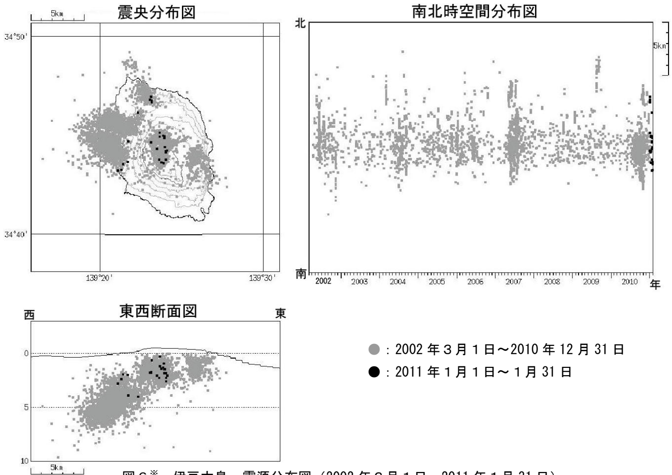
図 6 ※ 伊豆大島 震源分布図（2002 年 3 月 1 日～2011 年 1 月 31 日）
