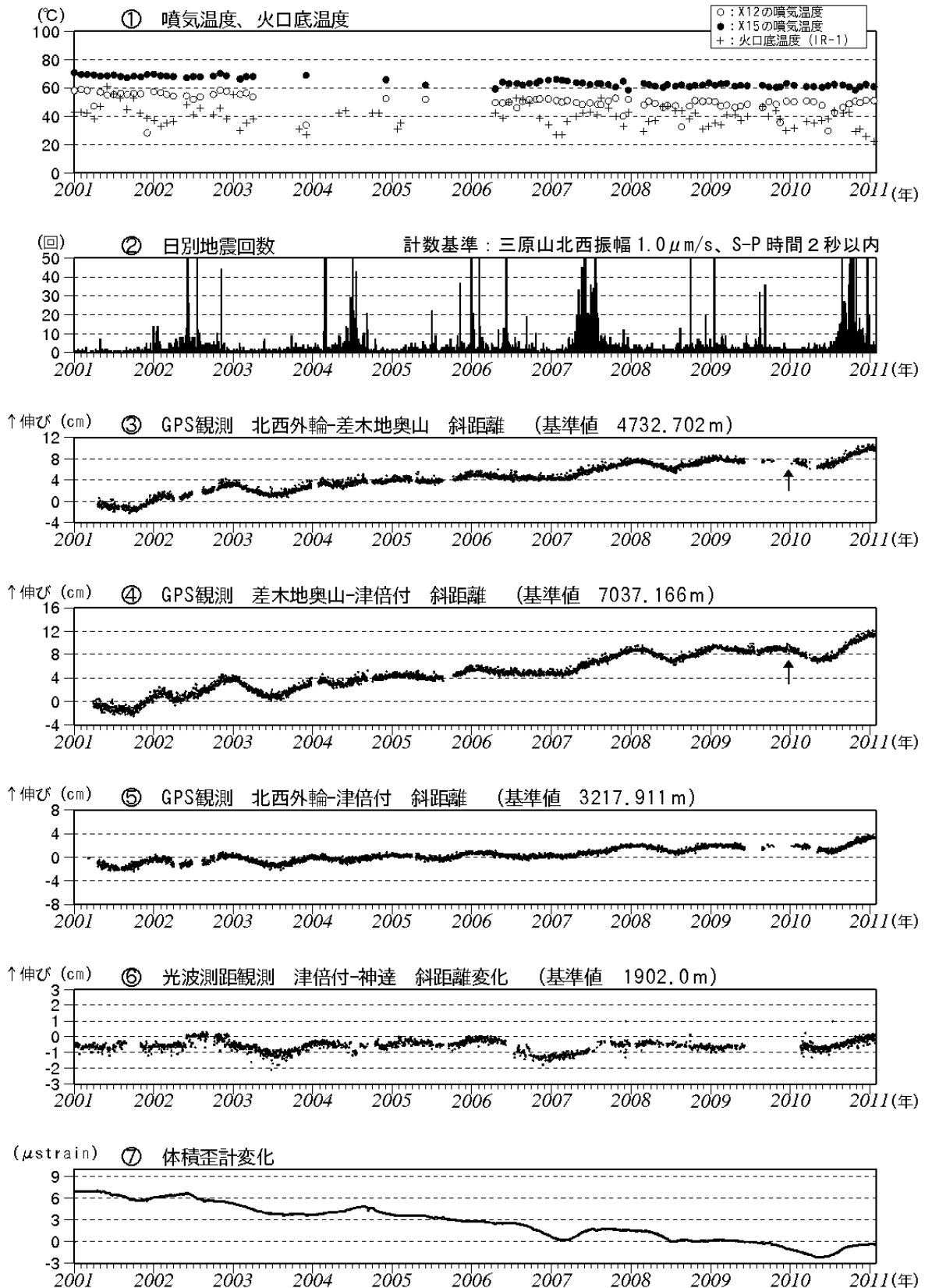
図 2 伊豆大島 最近の火山活動経過図（2001 年 1 月～2011 年 1 月）
