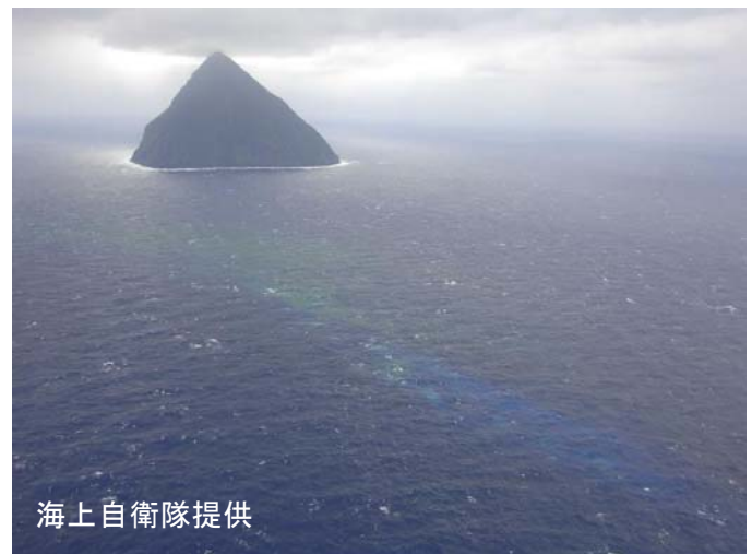
図 2※ 福徳岡ノ場 変色水の状況（12 月 18 日撮影）
