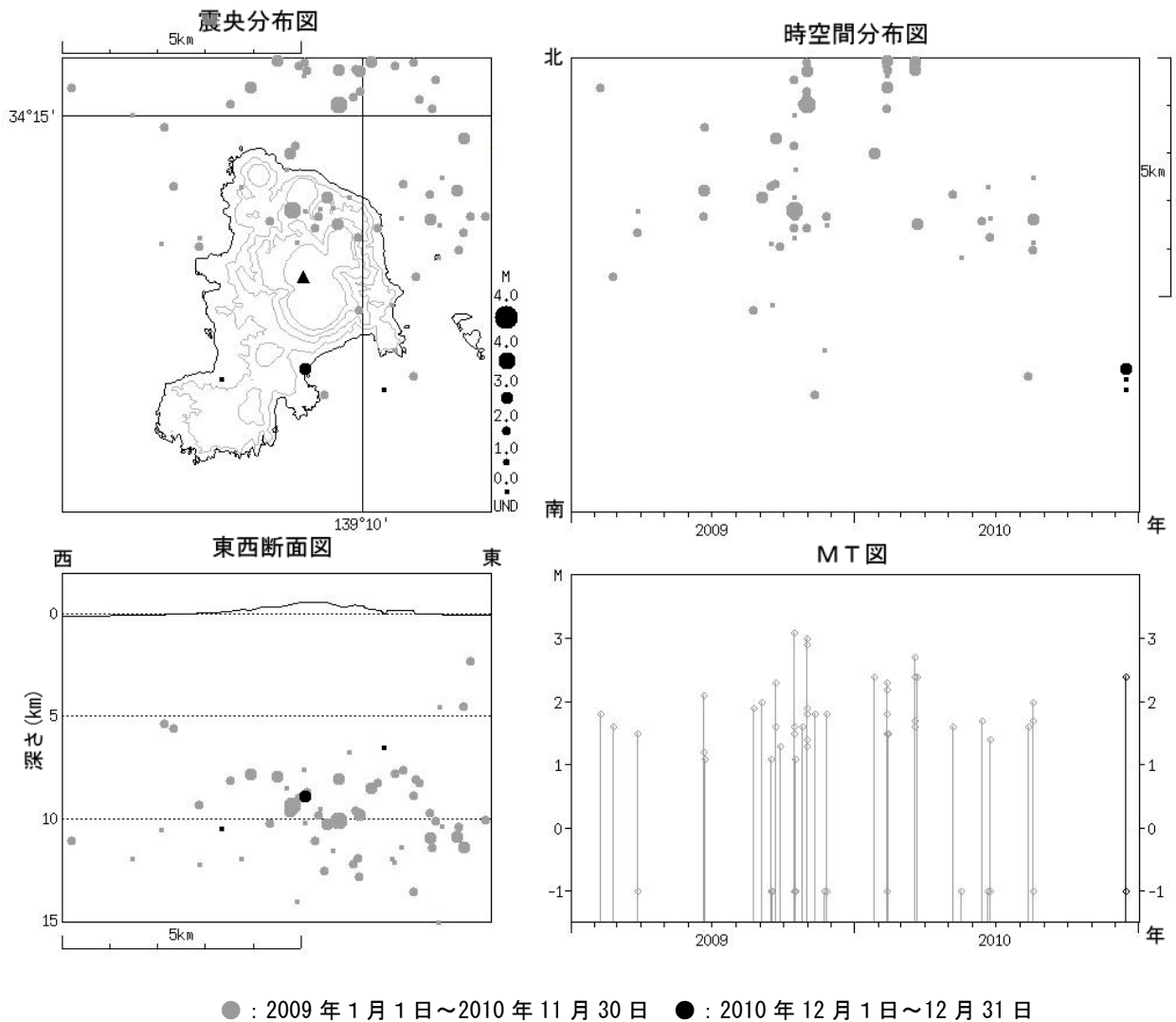
図 3※ 神津島 広域ネットによる山体・周辺の地震活動（2009 年 1 月 1 日～2010 年 12 月 31 日） M（マグニチュード）は地震の規模を表します。 図中の震源要素は一部暫定値が含まれており、後日変更することがあります。
