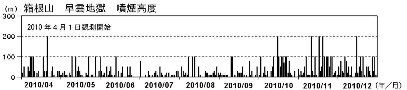
図 2 箱根山 早雲地獄の日別最大噴煙高度（2010 年 4 月 1 日～2010 年 12 月 31 日）
