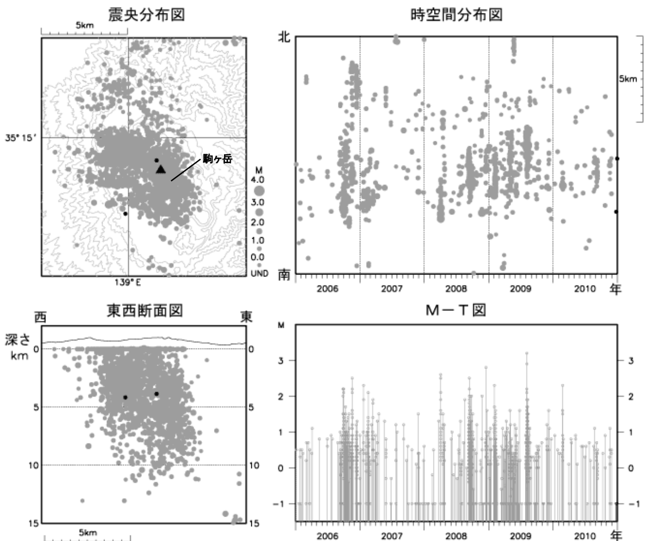
図 3※ 箱根山 震源分布図（2006 年 1 月 1 日～2010 年 12 月 31 日）
