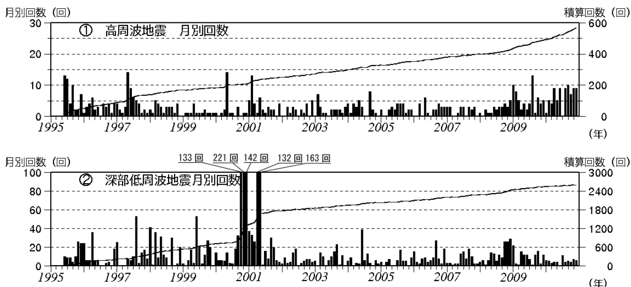
図 1 富士山 月別地震回数(1995 年 6 月～2010 年 12 月)
