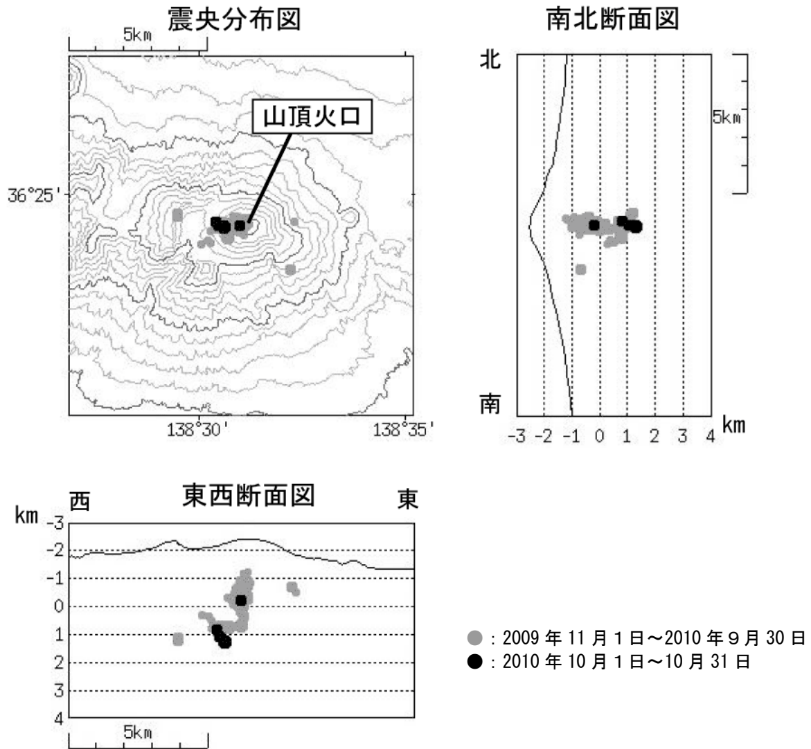
図 4 ※ 浅間山 震源分布図（2009 年 11 月 1 日～2010 年 10 月 31 日）
