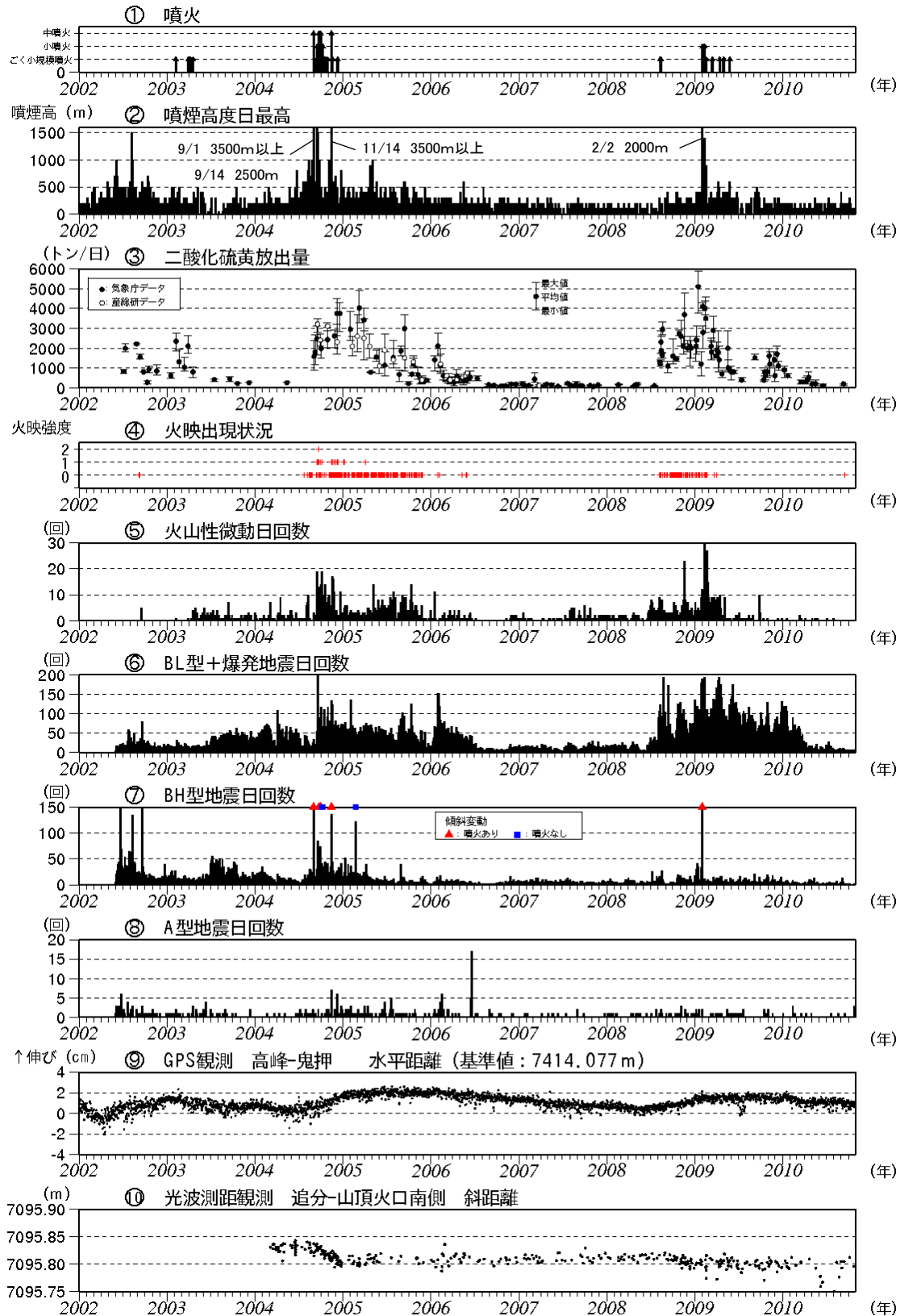
図 3※ 浅間山 最近の火山活動の推移（2002 年 1 月 1 日～2010 年 10 月 31 日）
