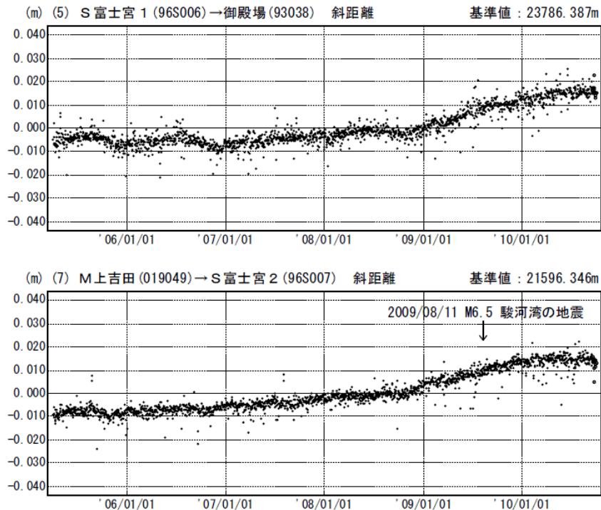
図 3※ 富士山 国土地理院による GPS 観測結果 1) （2005 年 4 月 1 日～2010 年 10 月 2 日）
