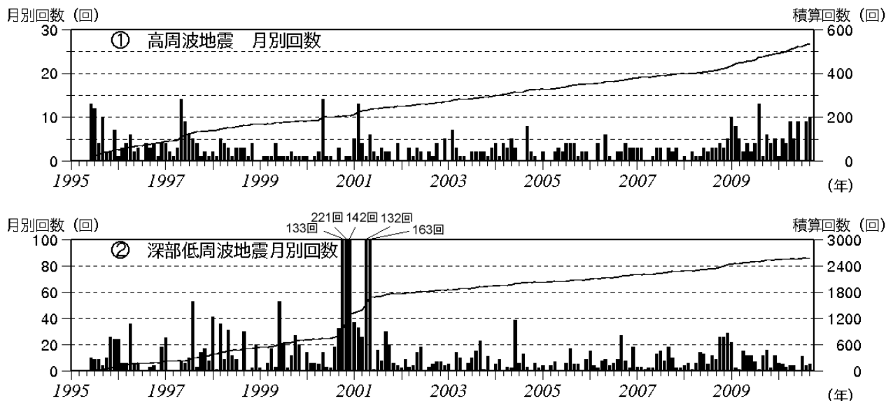
図 1※ 富士山 月別地震回数(1995 年 6 月～2010 年 9 月)
