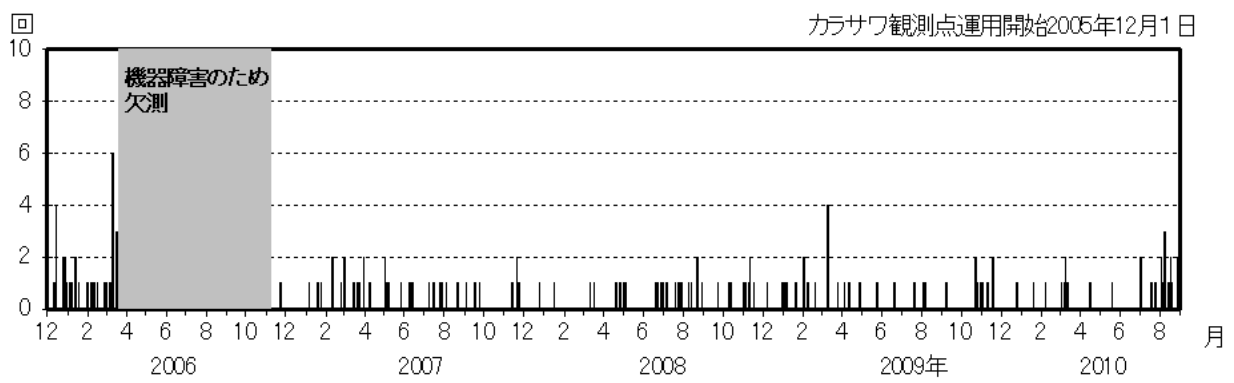
図 3 新潟焼山 日別地震回数（2005 年 12 月 1 日～2010 年 8 月 31 日）
