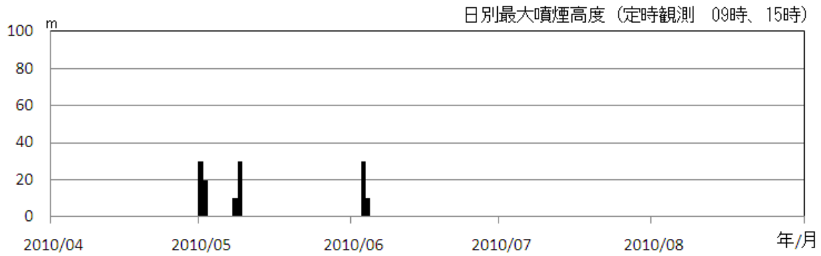
図 2 ※ 新潟焼山 日別最大噴気高度（2010 年 4 月 1 日～2010 年 8 月 31 日）
