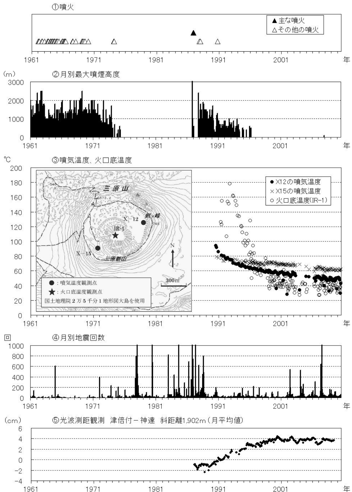
図4 伊豆大島 長期間の火山活動経過図（1961年1月～2010年7月）
