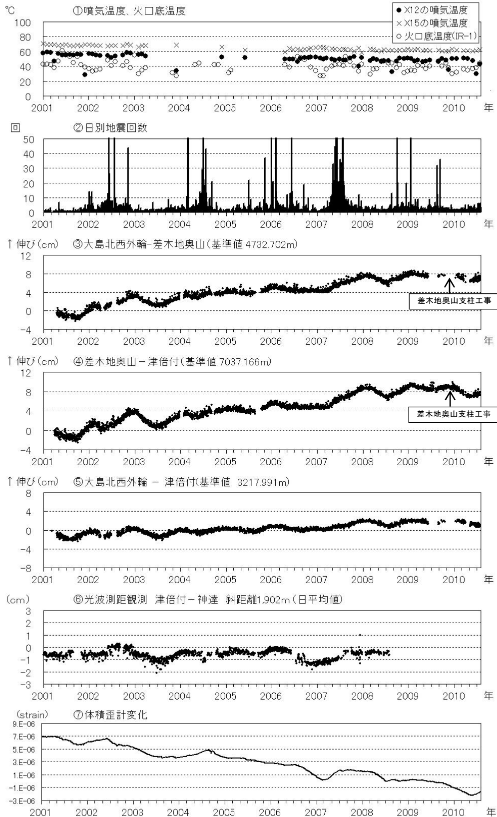
図5 伊豆大島 最近の火山活動経過図（2001年1月～2010年7月）
