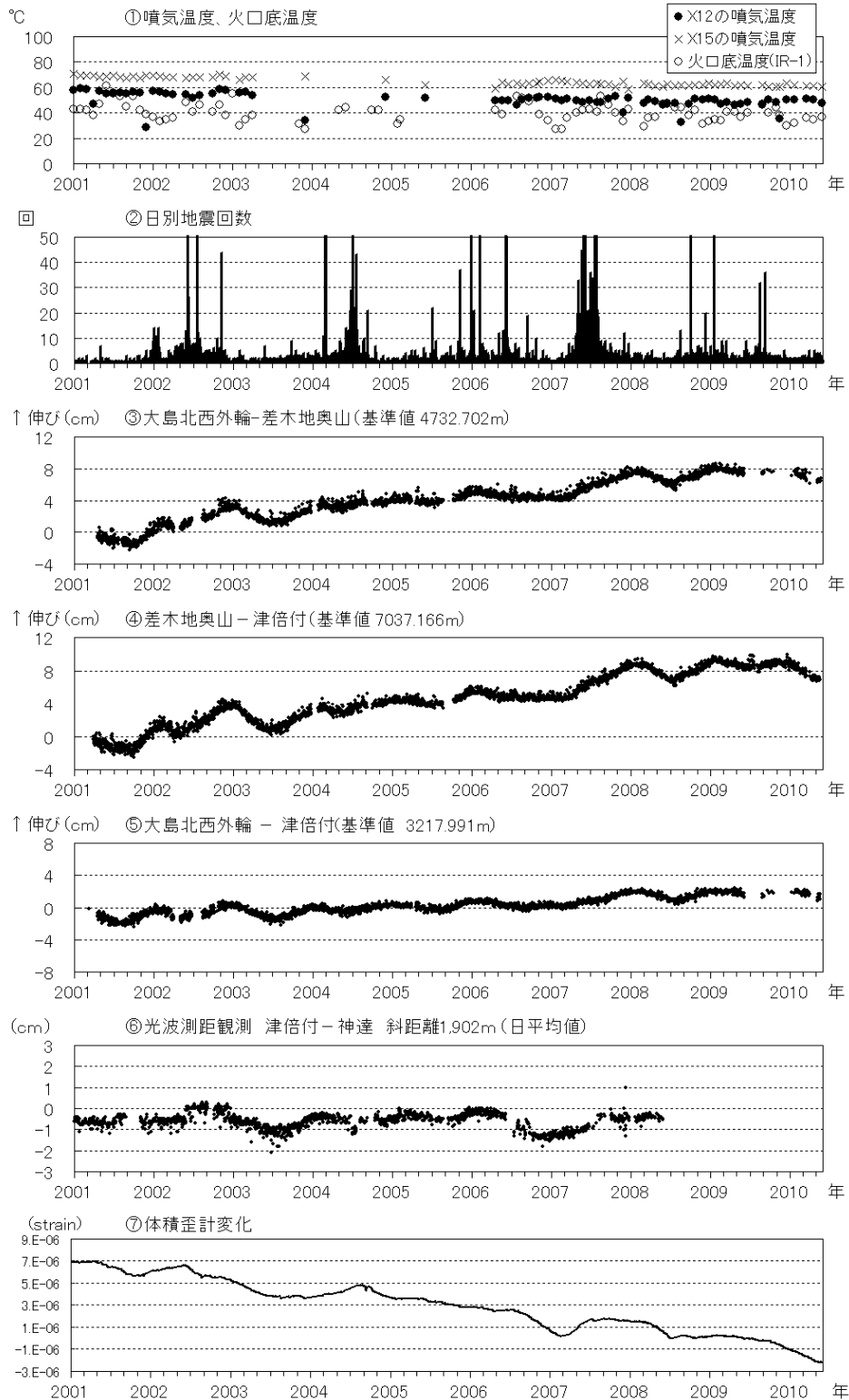
図5 伊豆大島 最近の火山活動経過図 (2001年1月~2010年5月)
