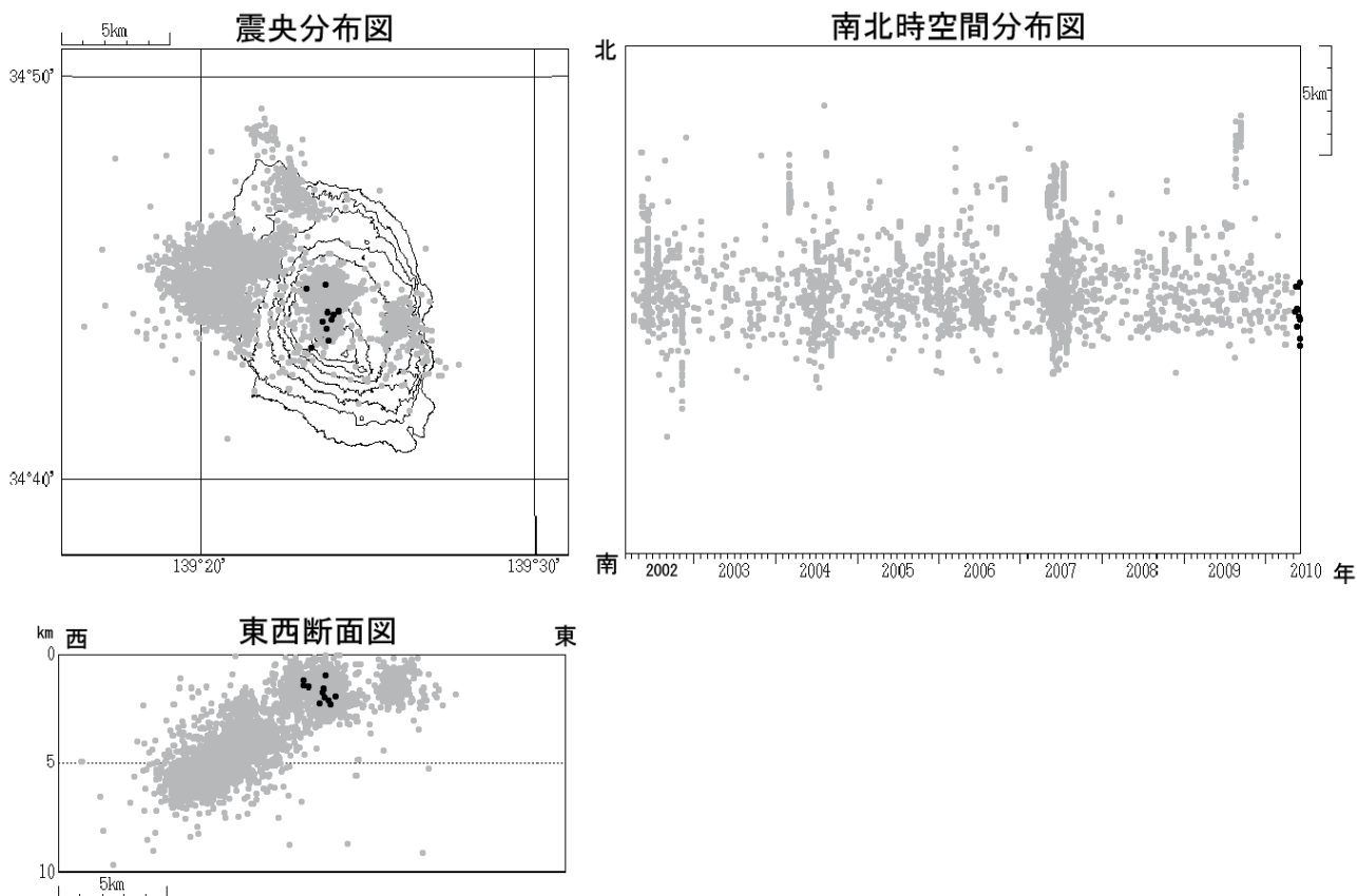
図 6※ 伊豆大島 震源分布図 (2002 年 3 月 1 日～2010 年 5 月 31 日)
