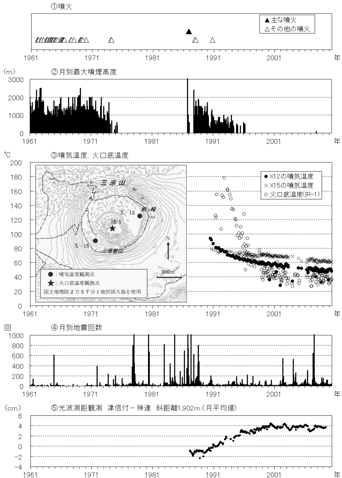
図4 伊豆大島 長期間の火山活動経過図（1961年1月～2010年5月）
